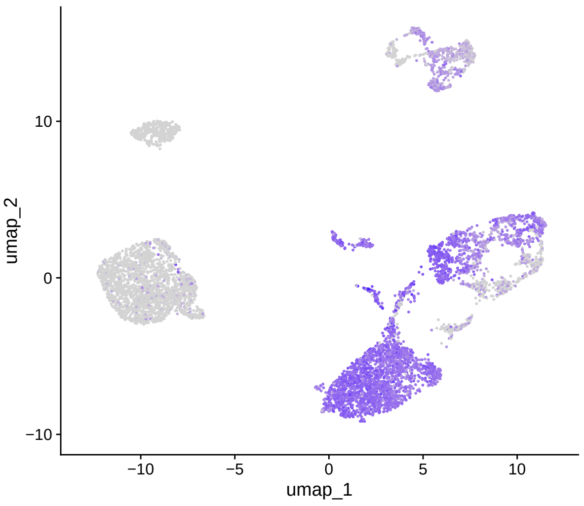
HLA-DPA1
