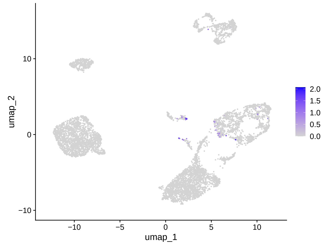
ITGAX
