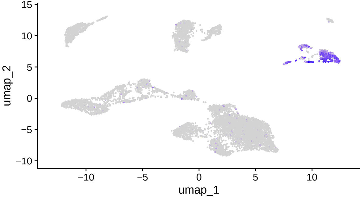
LYZ
