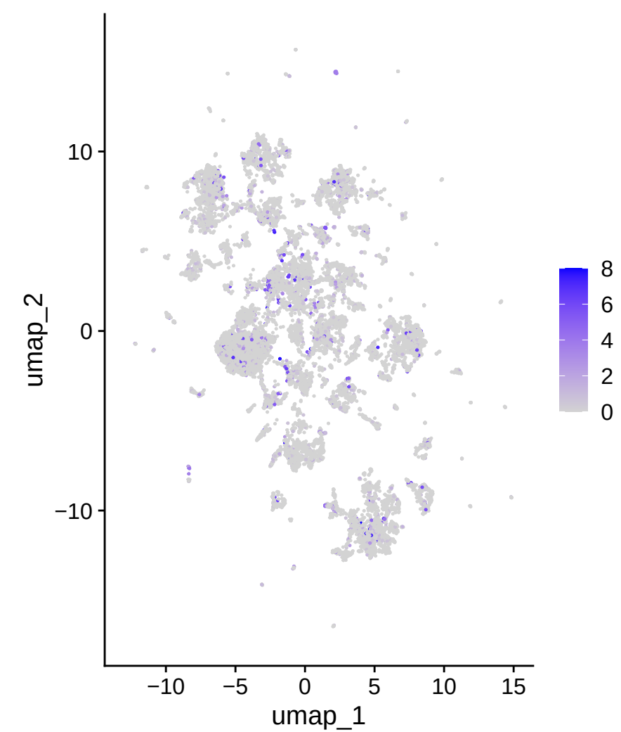
IGHA1
