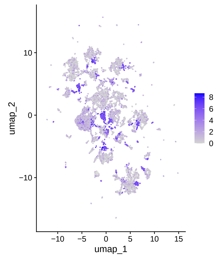
IGHG2
