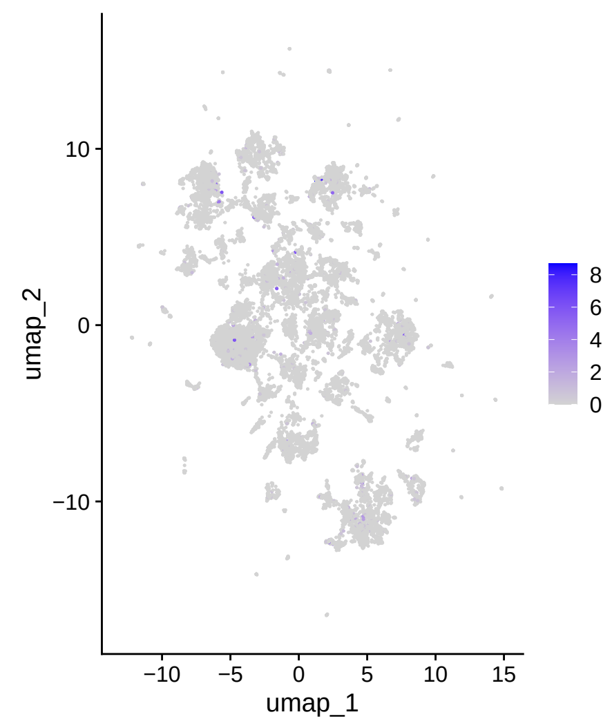
IGHE
