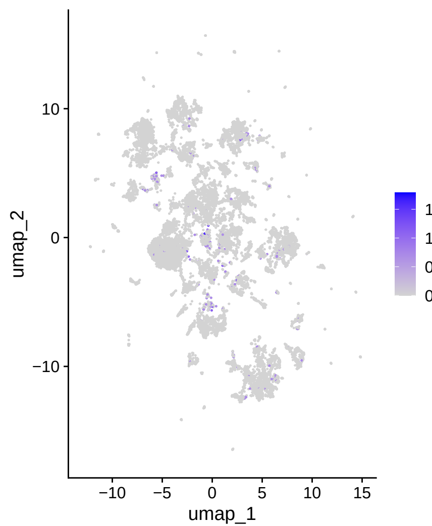
IGHG3
