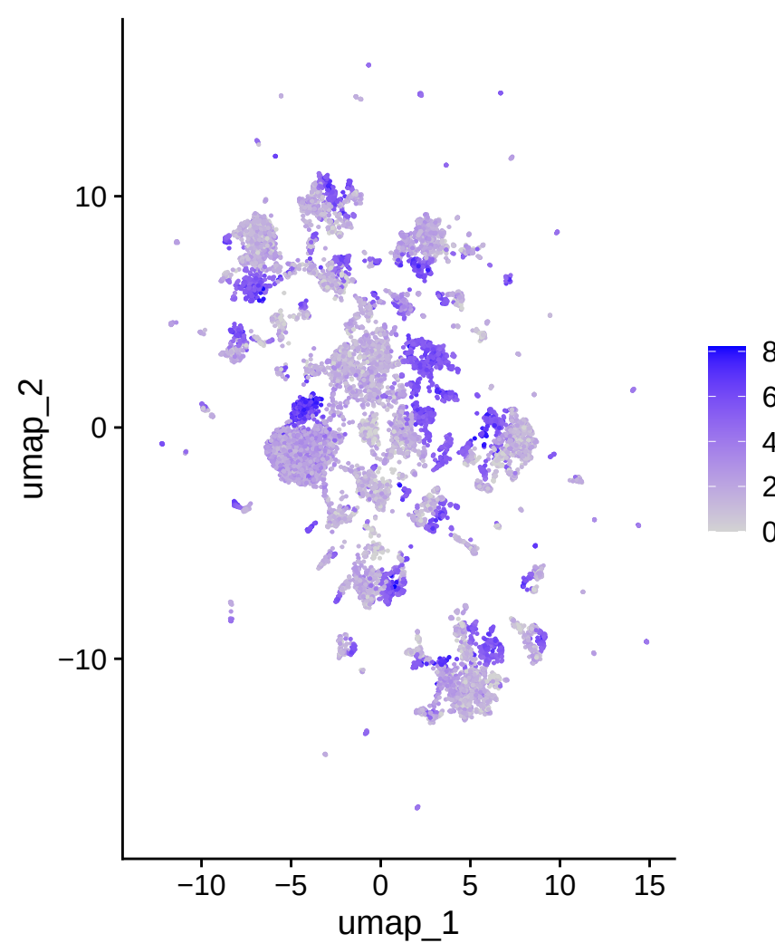
IGHA2
