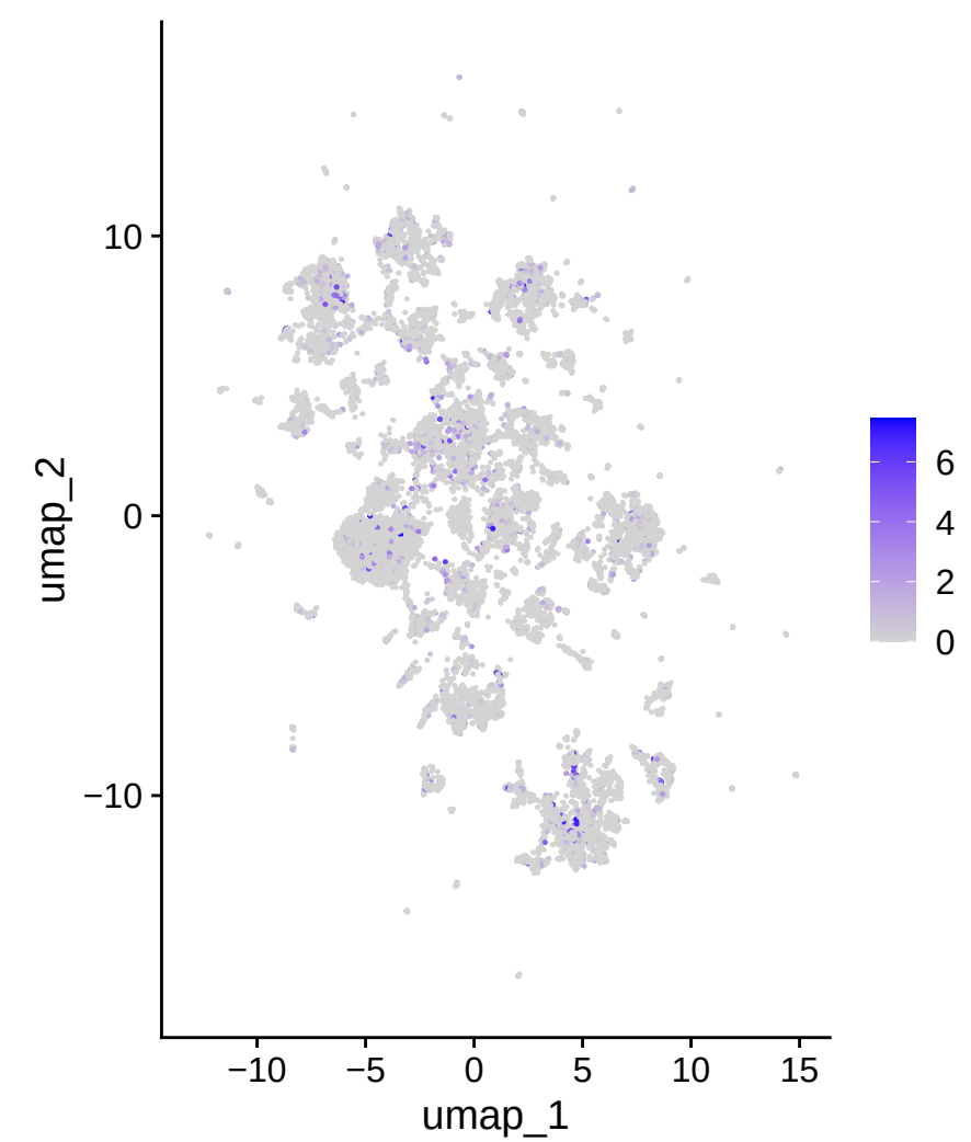
IGHG4
