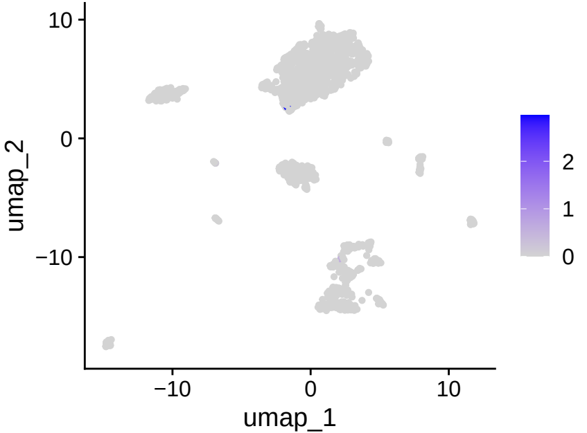
CD8A
