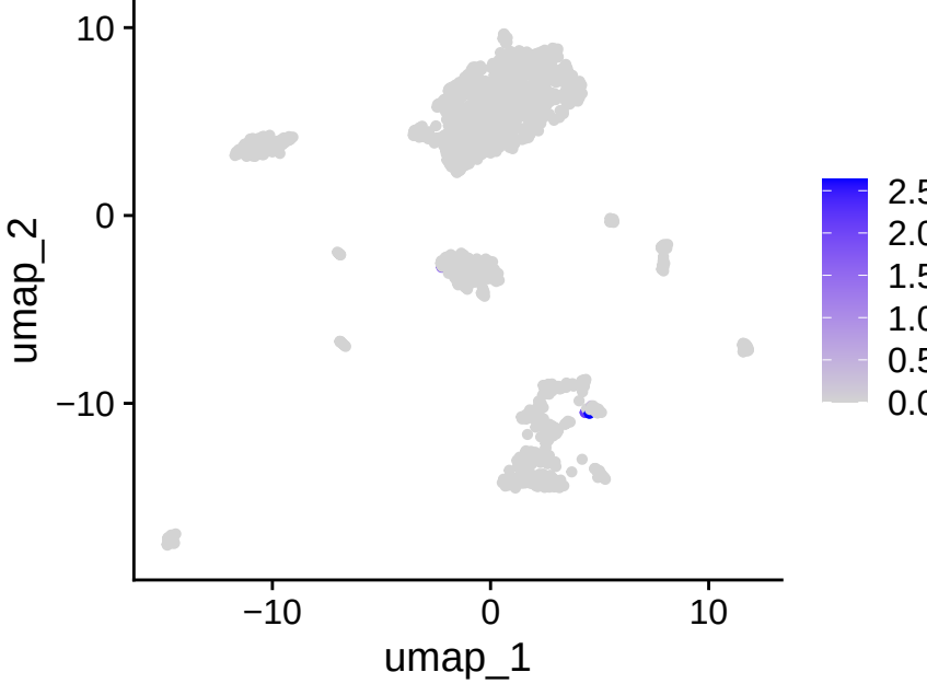
CD8A
