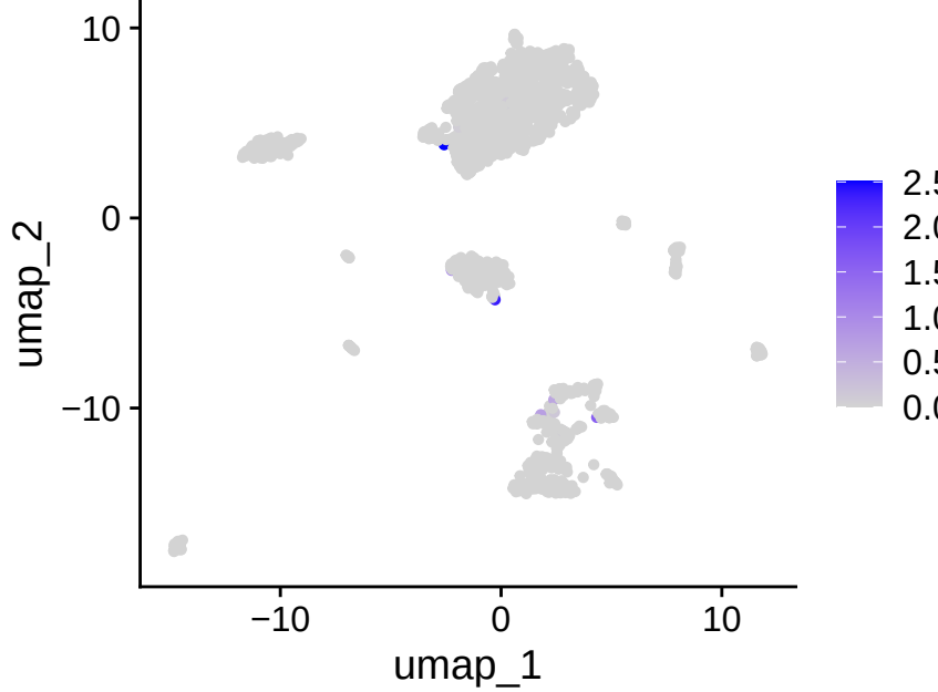
CD2
