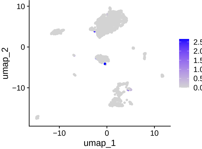
TRBC1
