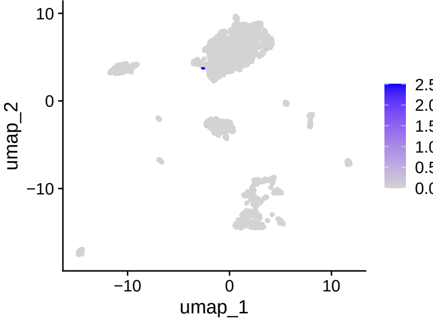
CD4
