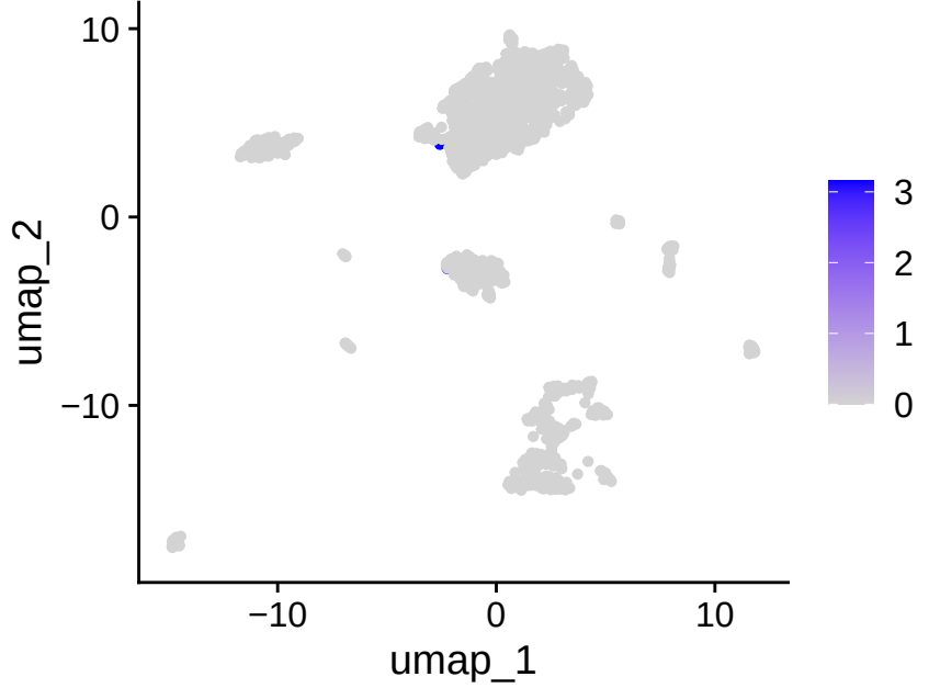
CD2
