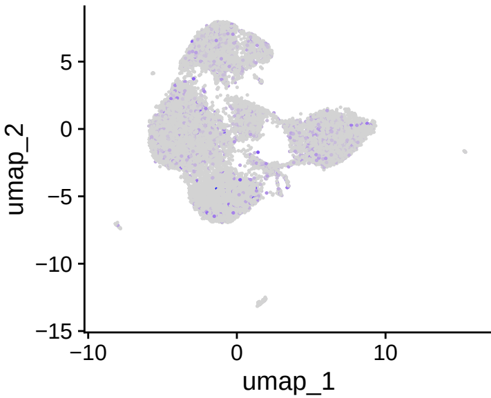
PCNA
