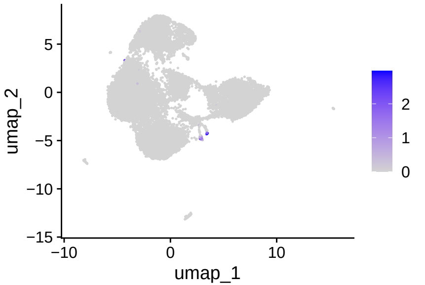
CXCR4
