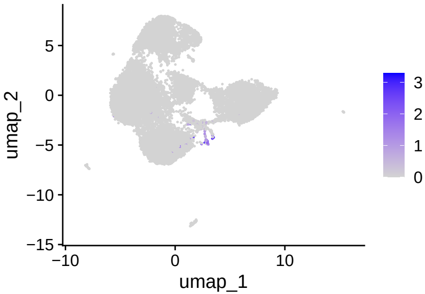
MME
