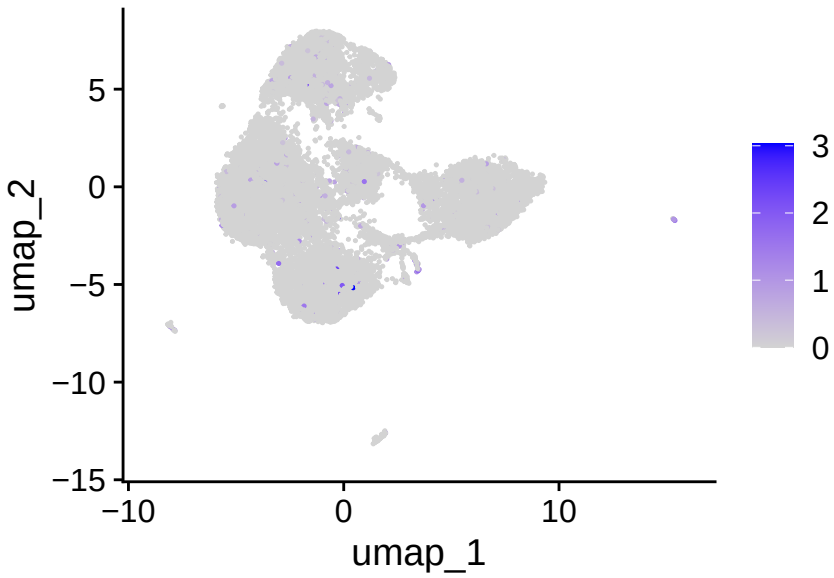
CD27
