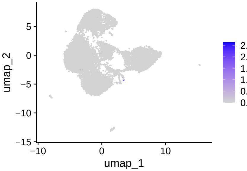
CD83
