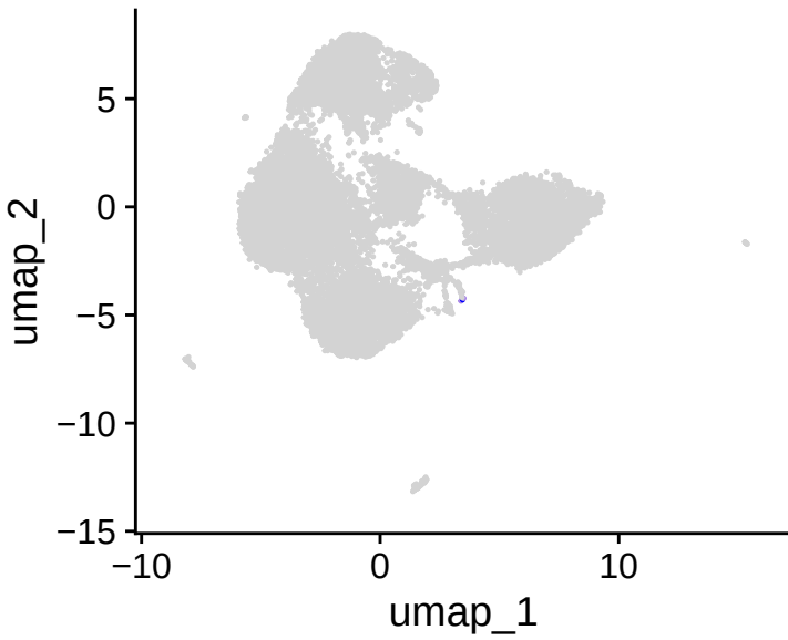
SERPINA9
