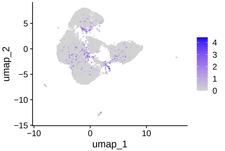
TCL1A
