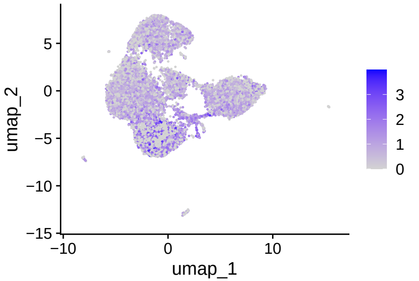
LMO2
