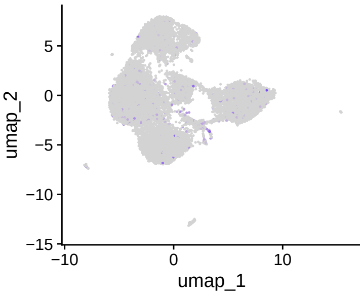
CD86
