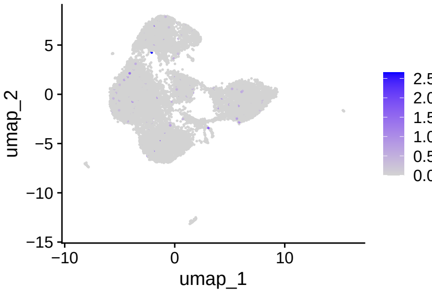
CD27
