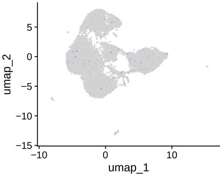
IL4R
