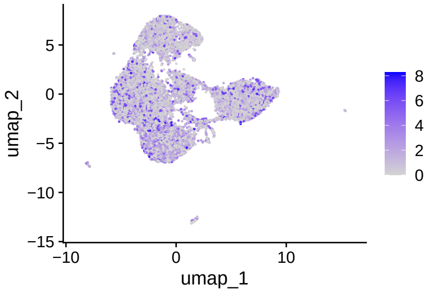
CD24
