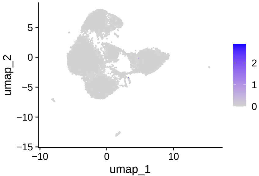
CD200
