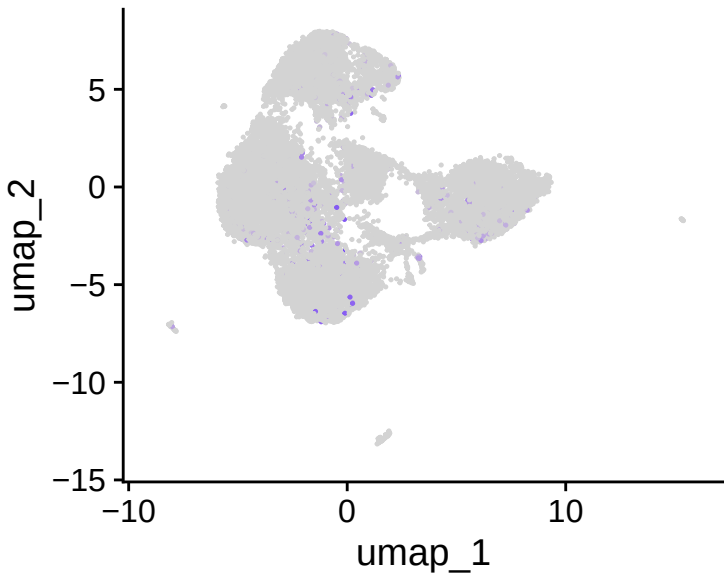
CD38
