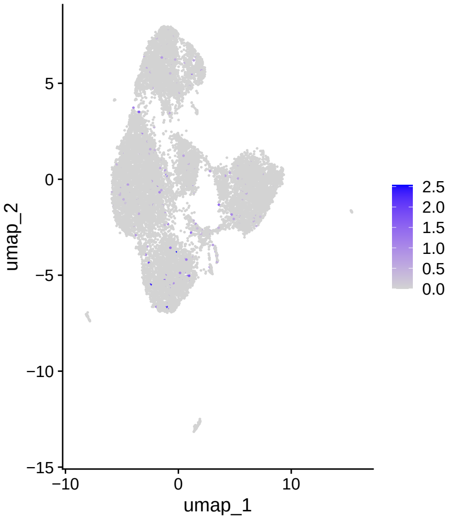
ITGAX
