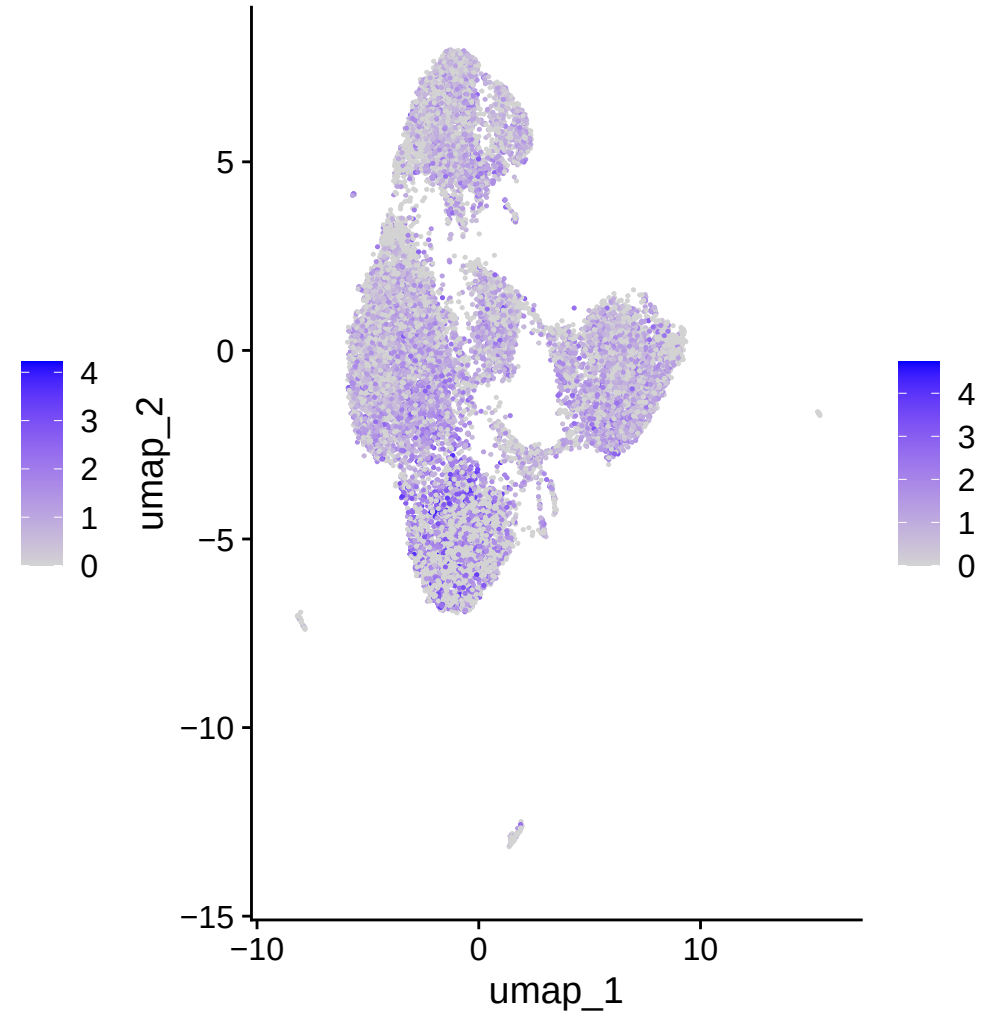
IRF4
