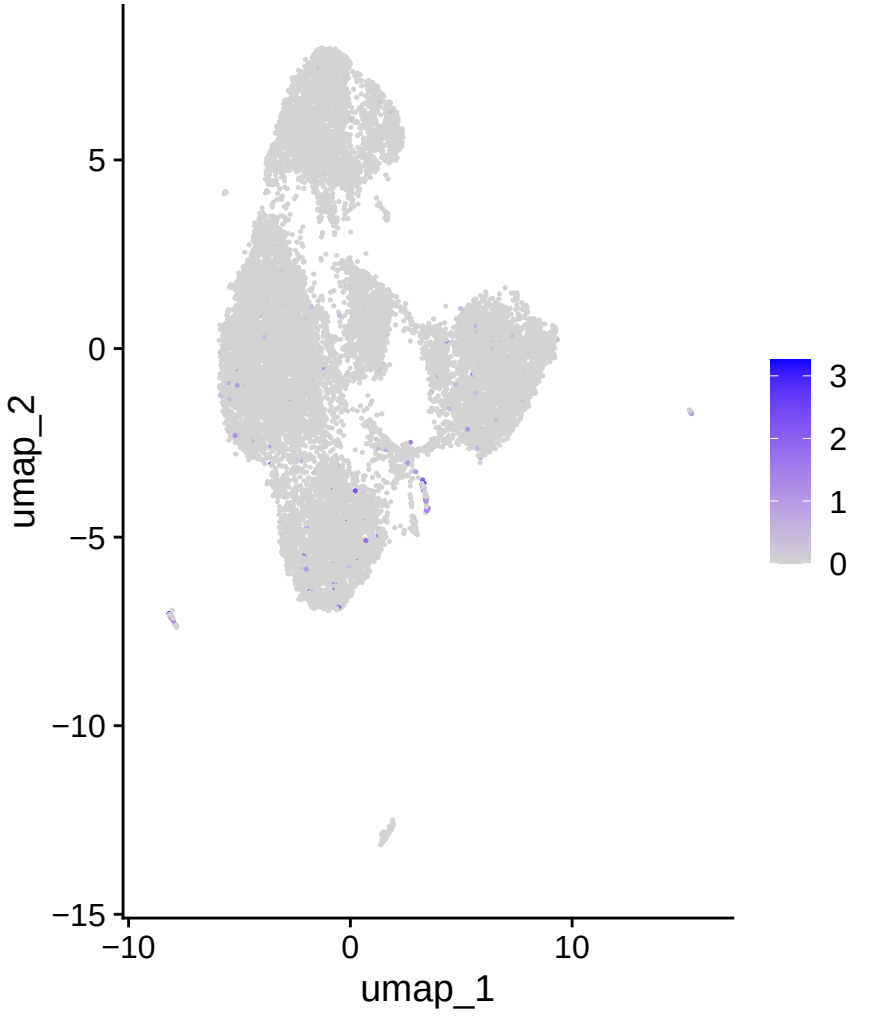
IRF8
