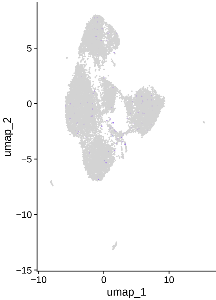
TBX21
