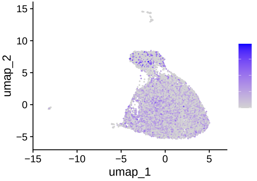
CD38
