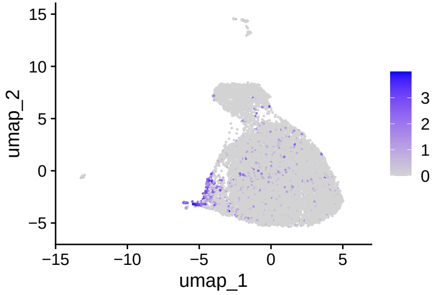
CD27
