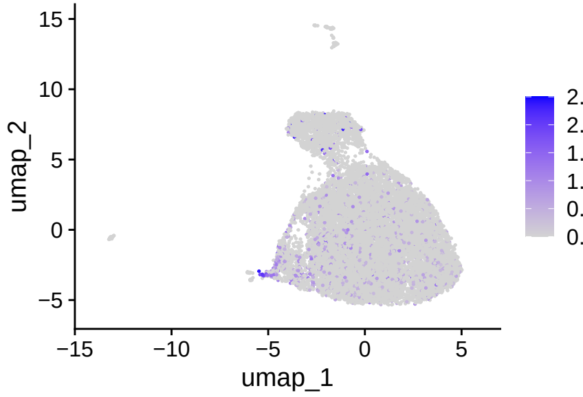
CXCR4
