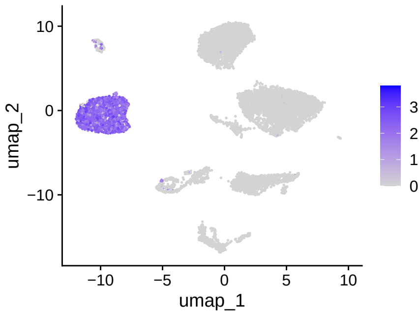
TRBC1
