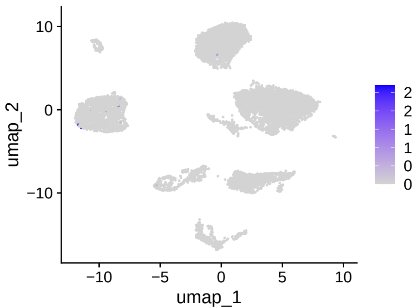
CD8A
