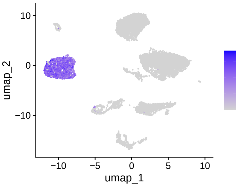
CD4
