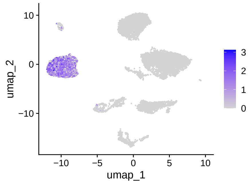
CD2
