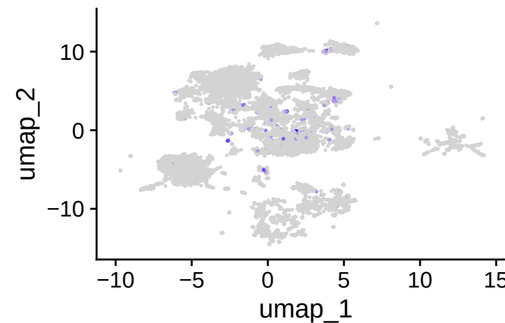
LYZ
