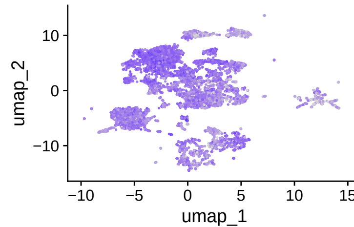
ITGAX
