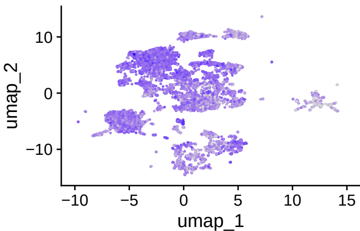
CD86
