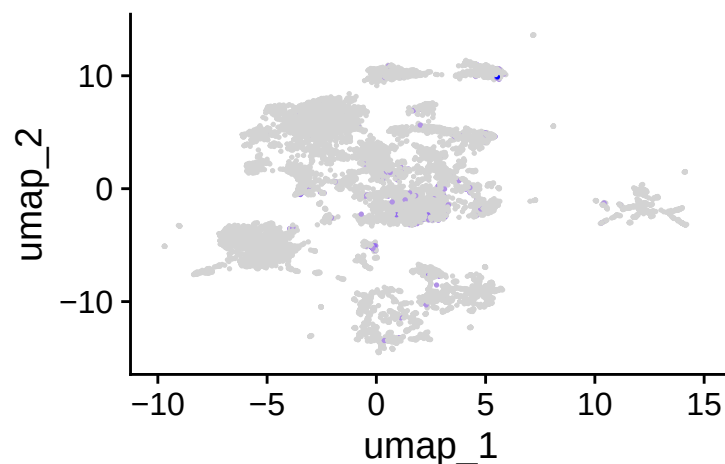
FLT3
