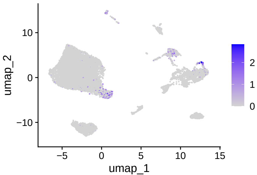
CD200
