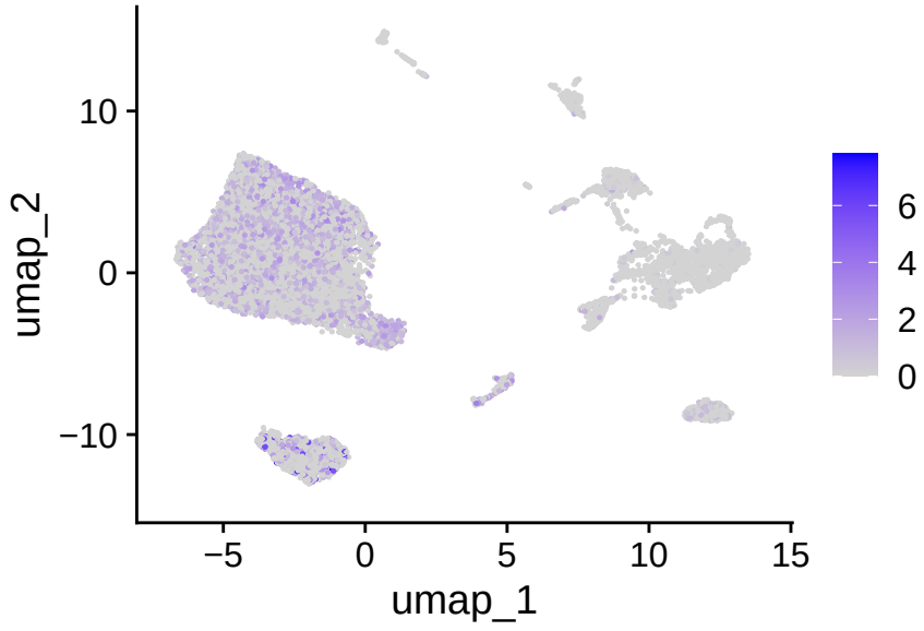
CD24
