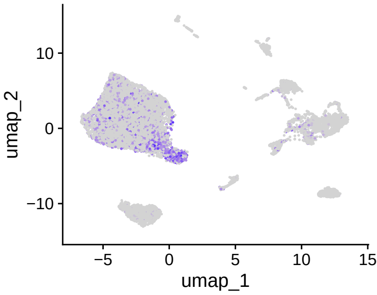
IL4R
