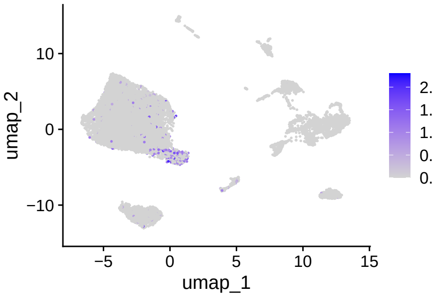
CD27
