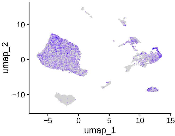
CD38
