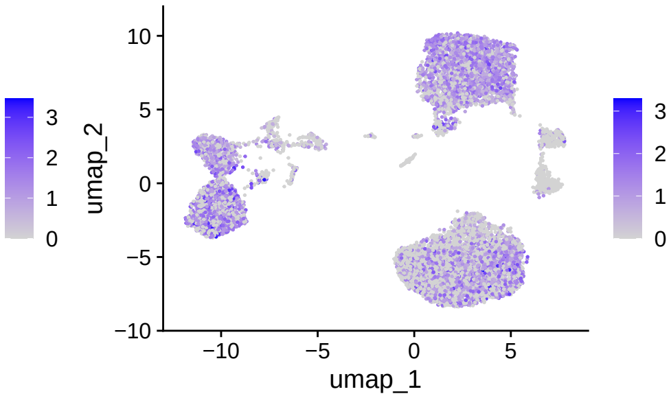
CD200
