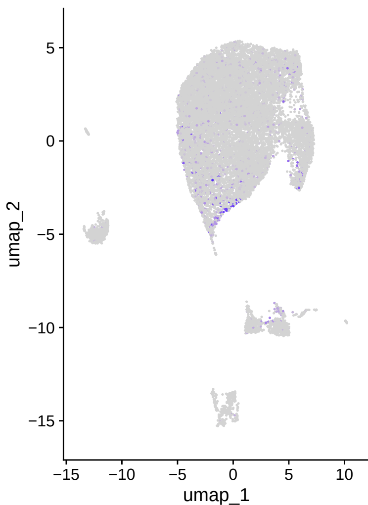
IGHA2
