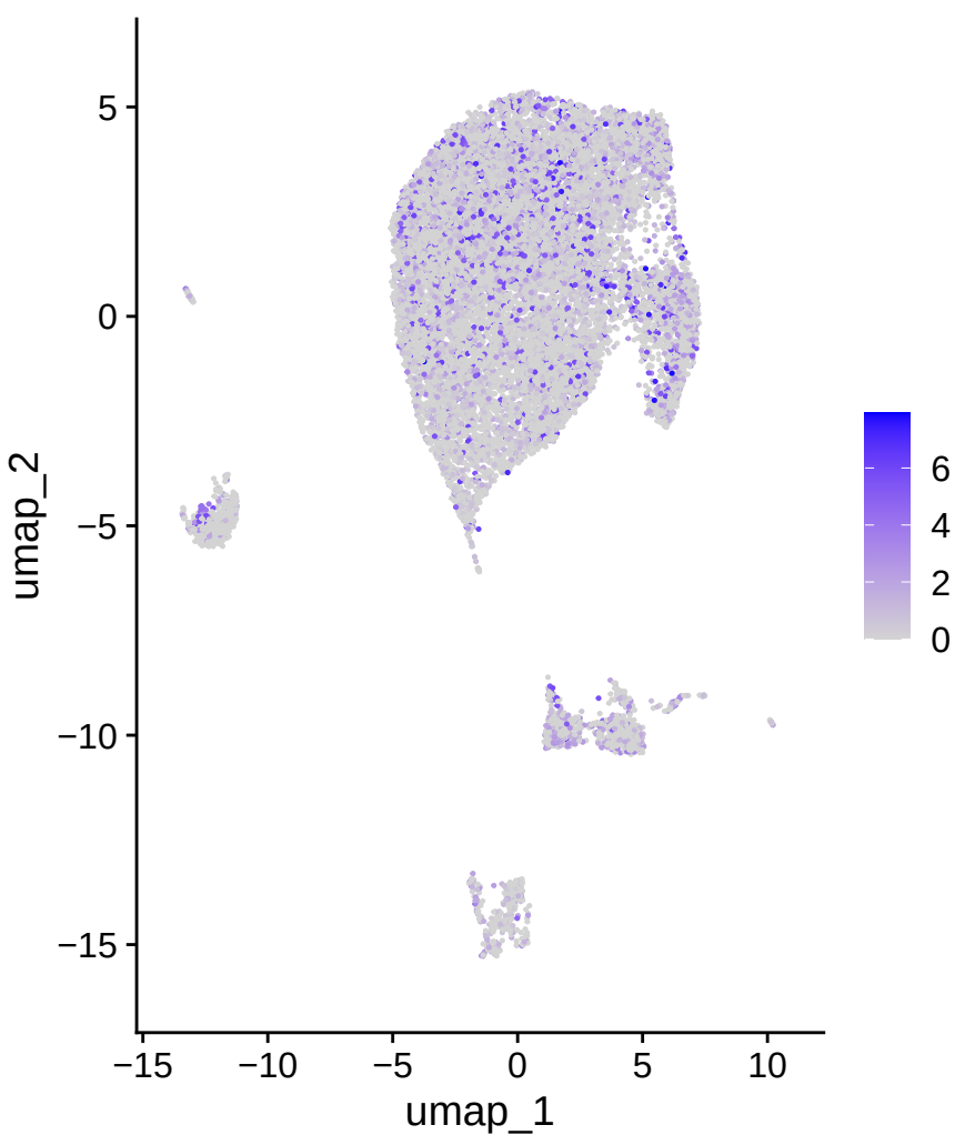
IGHG2
