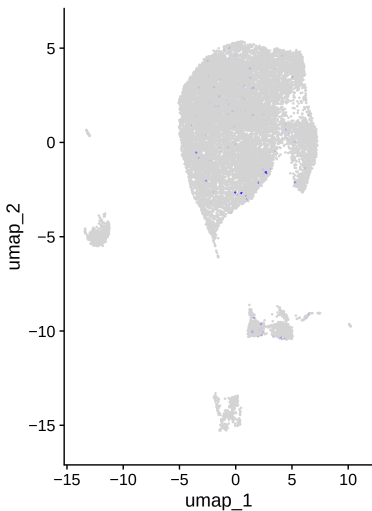
IGHG3
