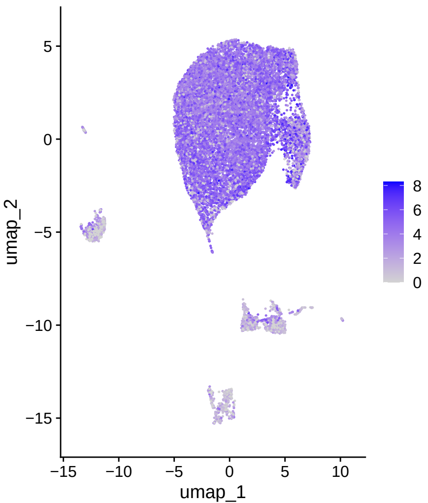
IGHA1
