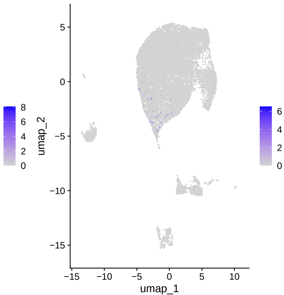
IGHE
