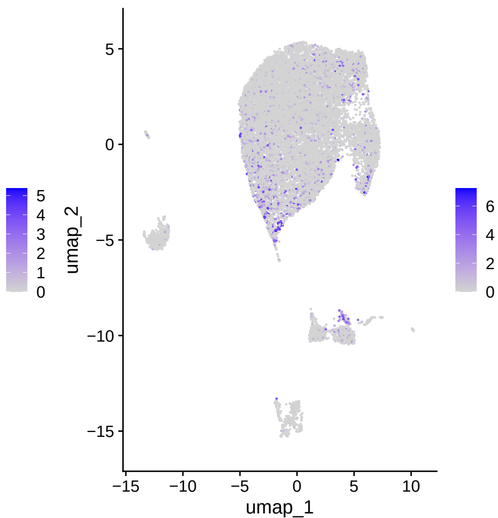
IGHG4
