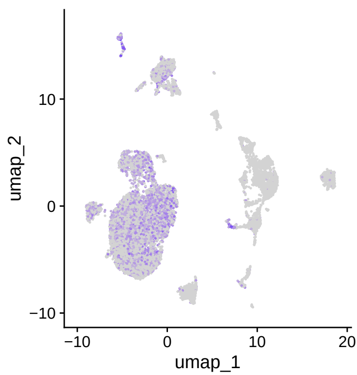
RORA
