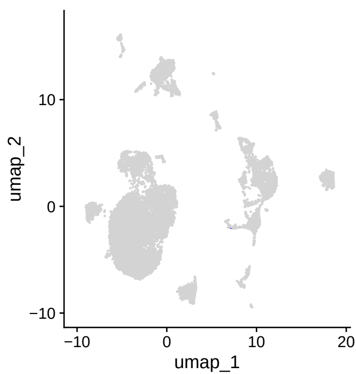
CD200
