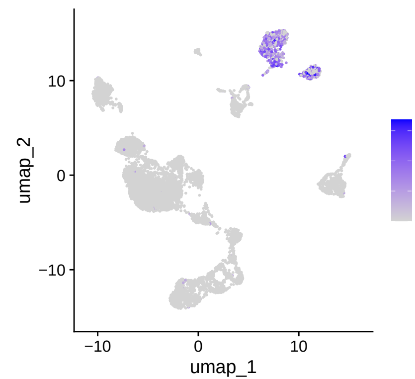
IL21
