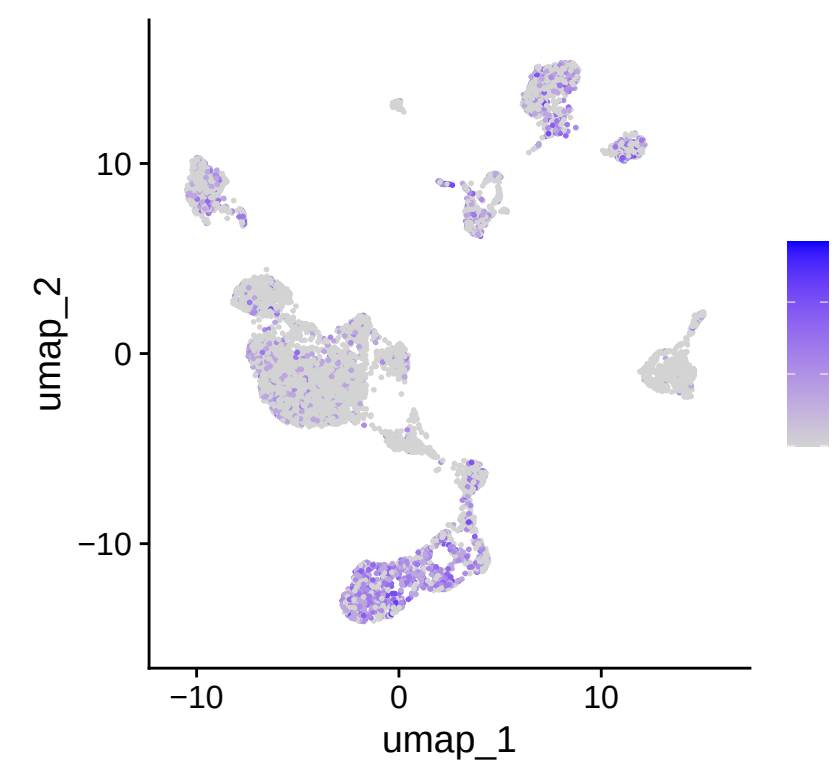
ICOS
