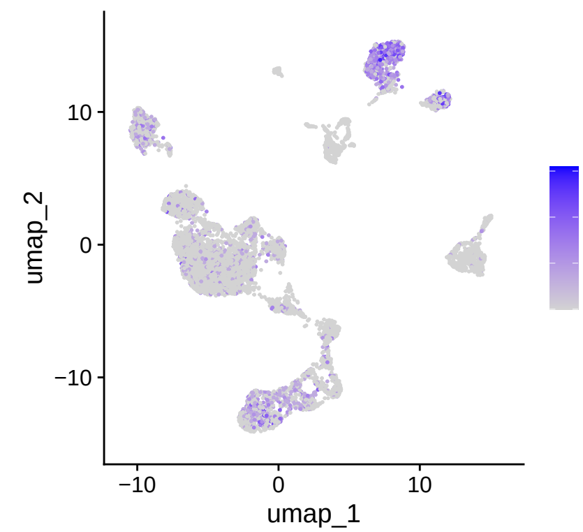
SLAMF6
