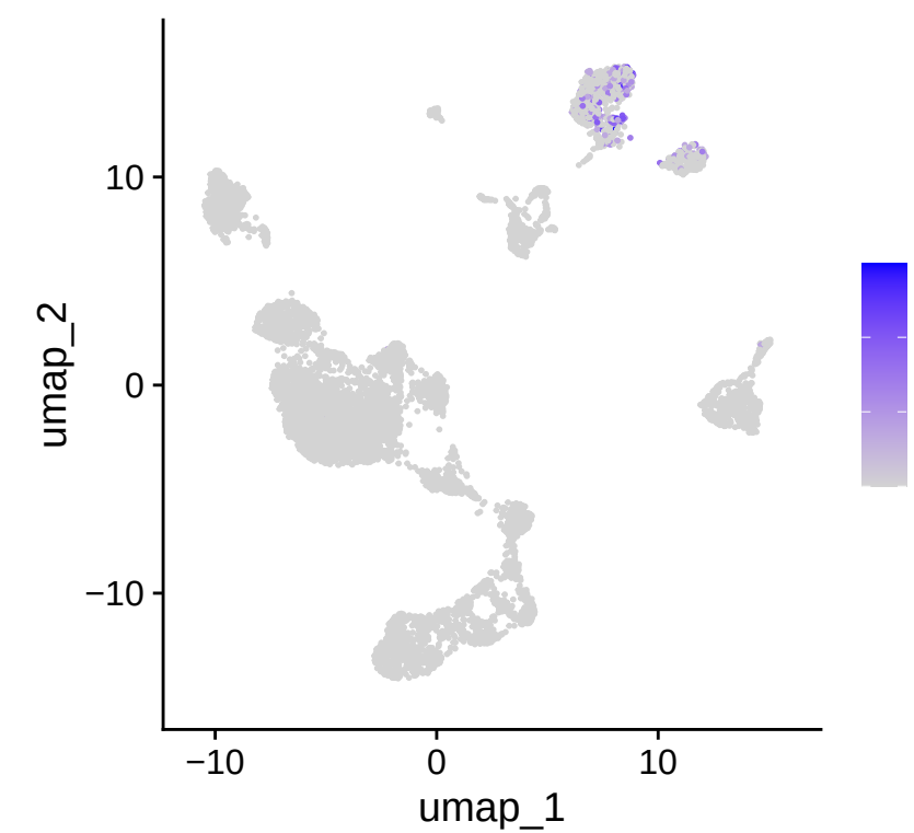
SLAMF6
