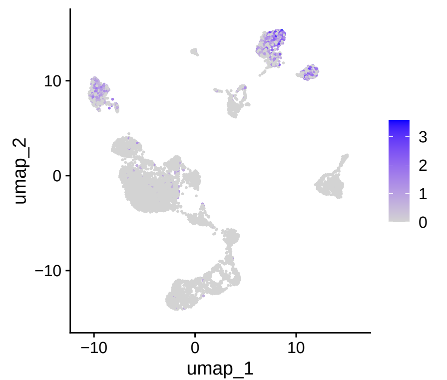
RORA
