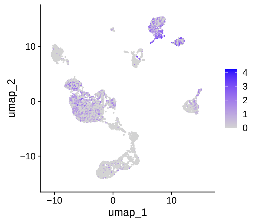
RORA
