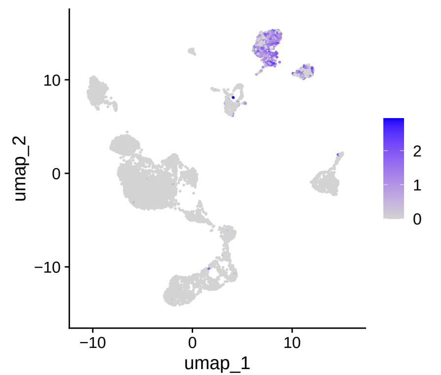
CD200
