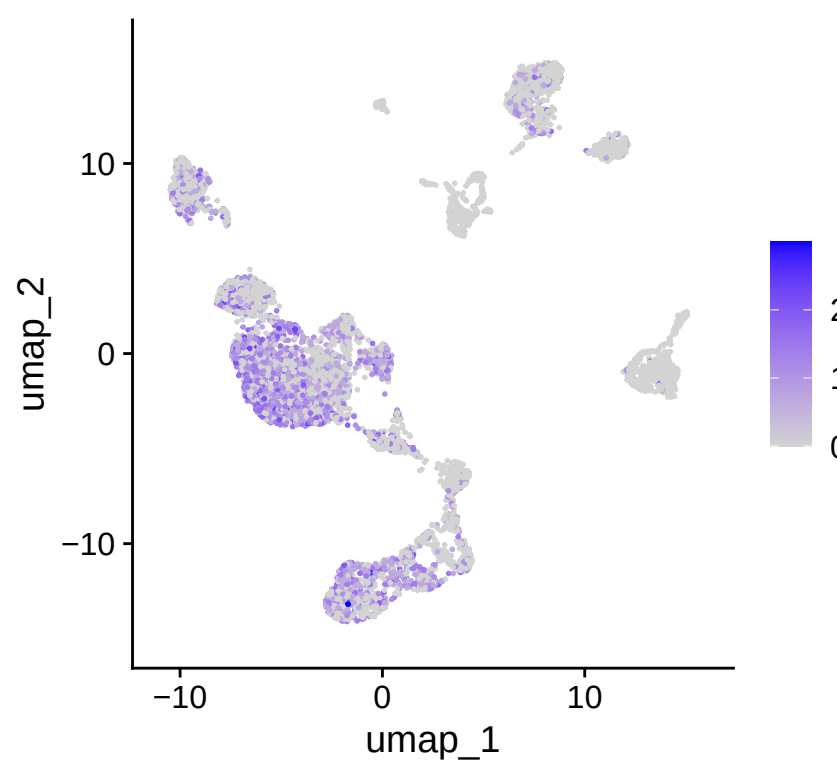
CD40LG
