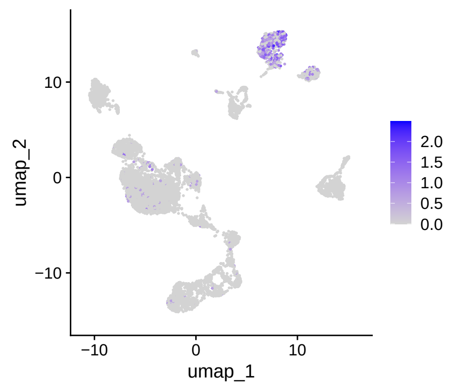
MAF
