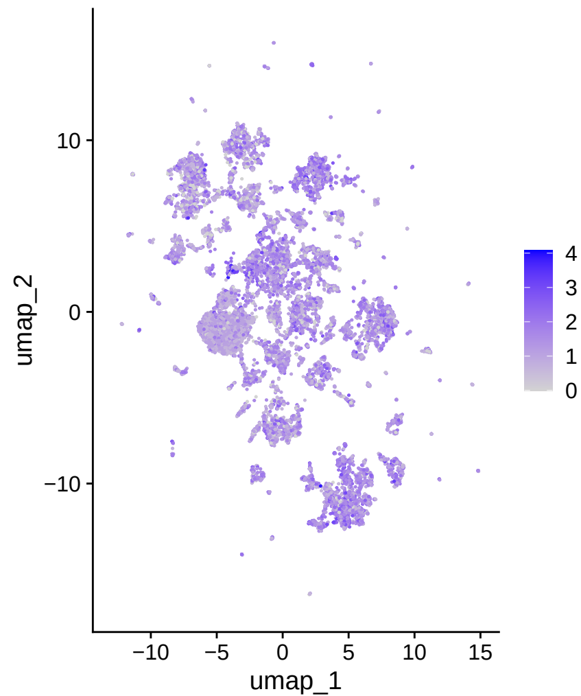
CD40
