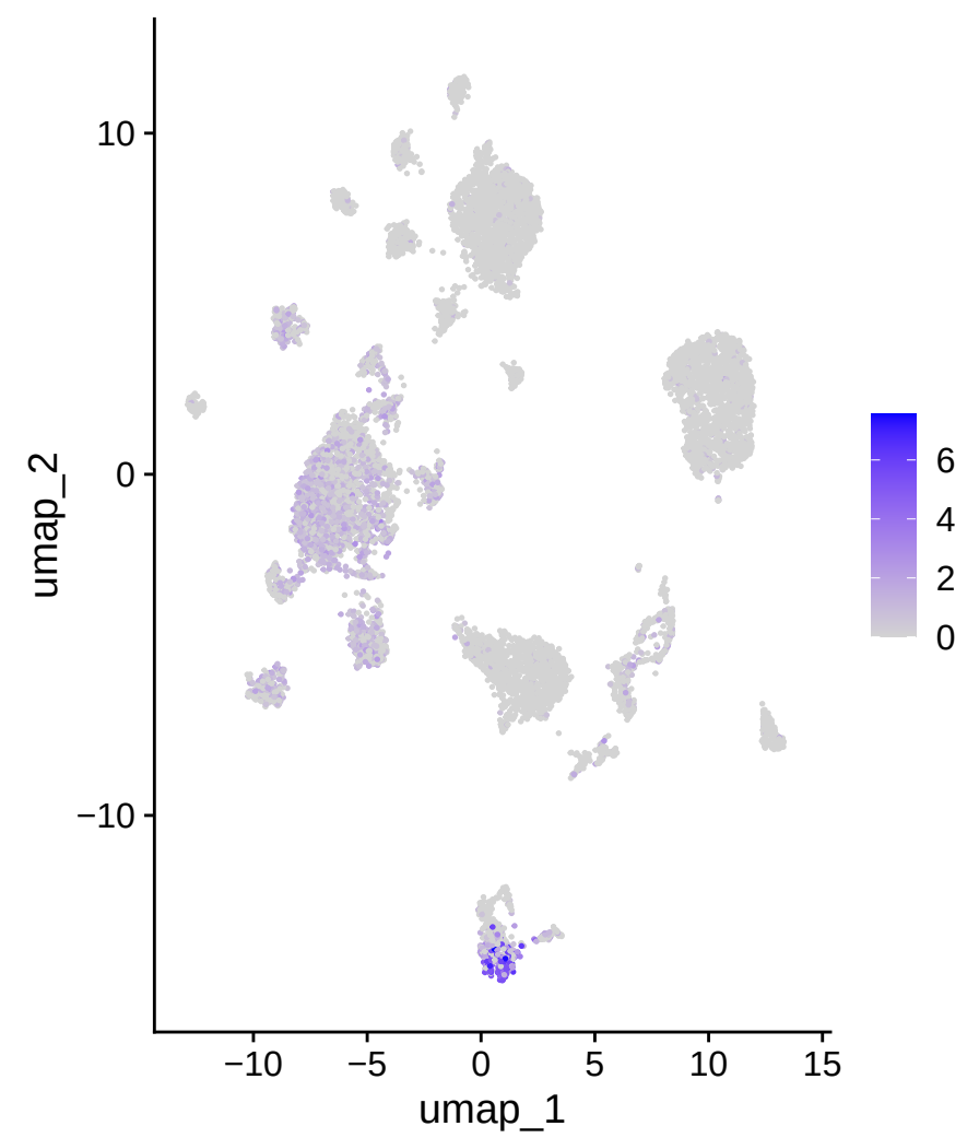
IGHA2
