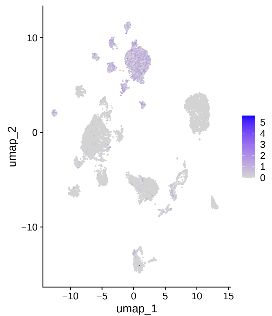
IGHG3
