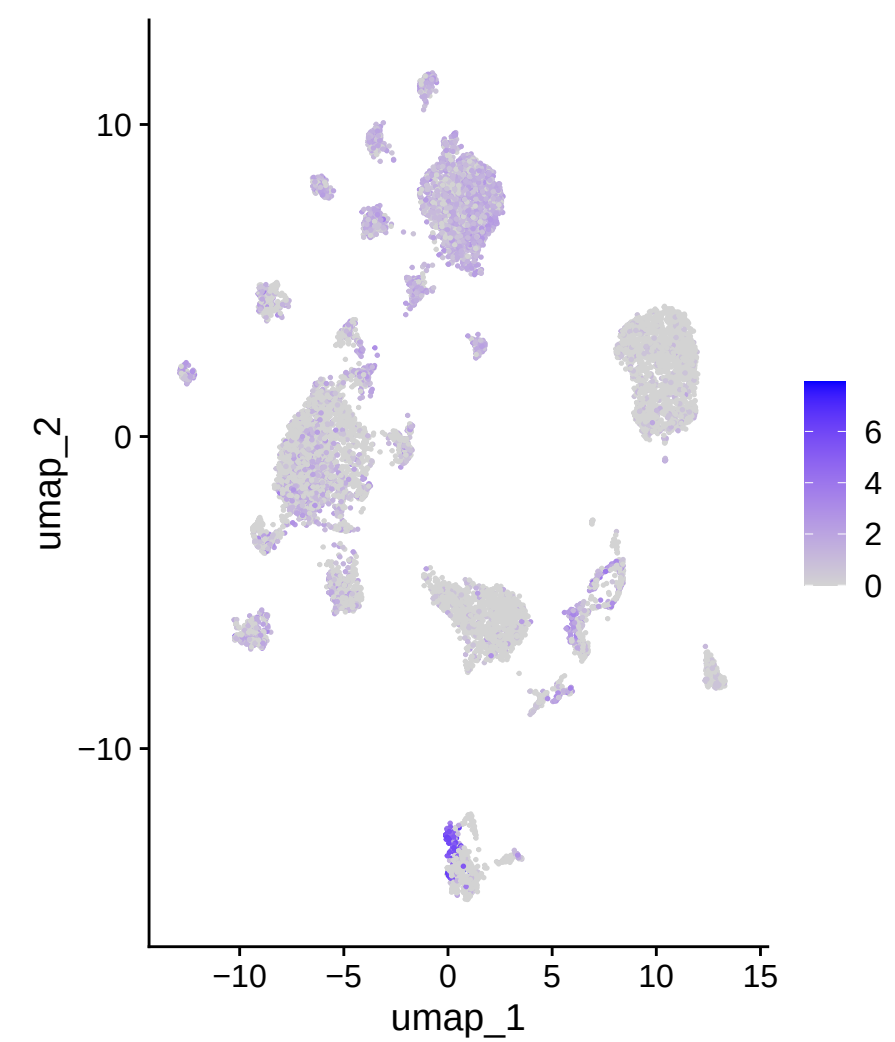
IGHG2
