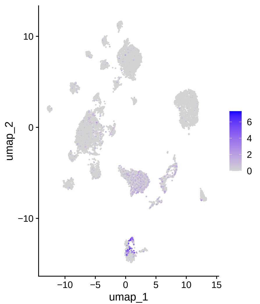
IGHG4
