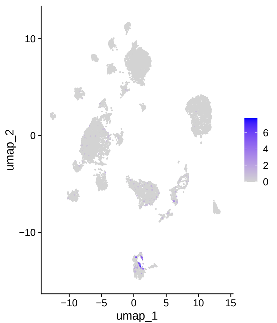
IGHE
