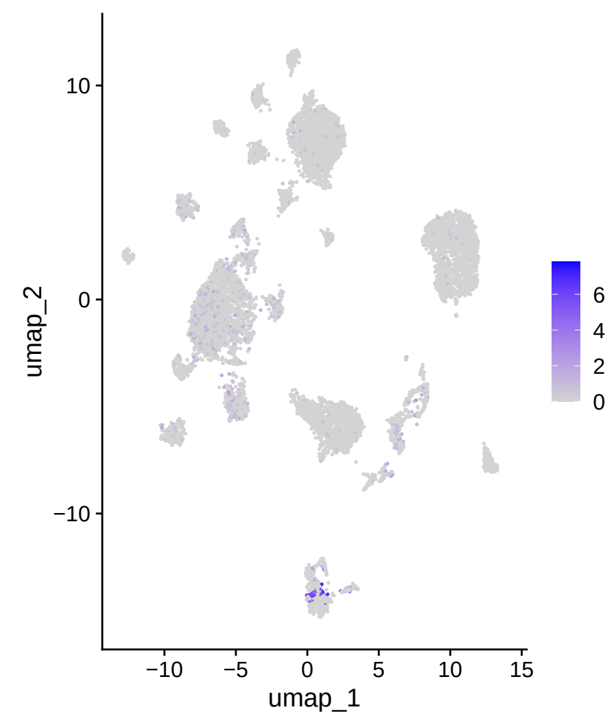
IGHA1
