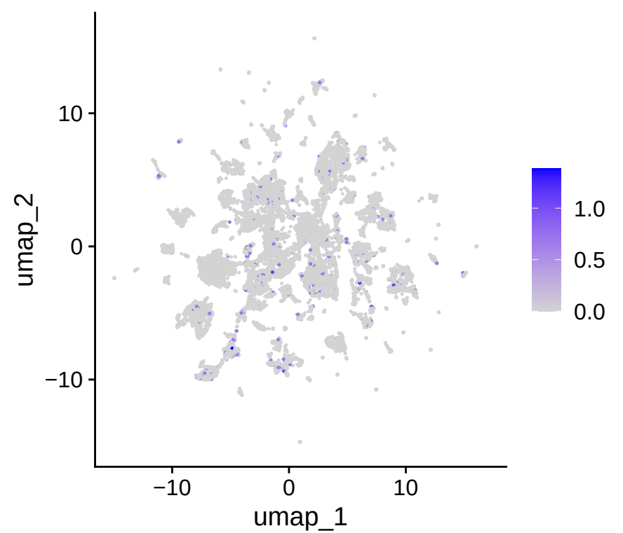
SLAMF6
