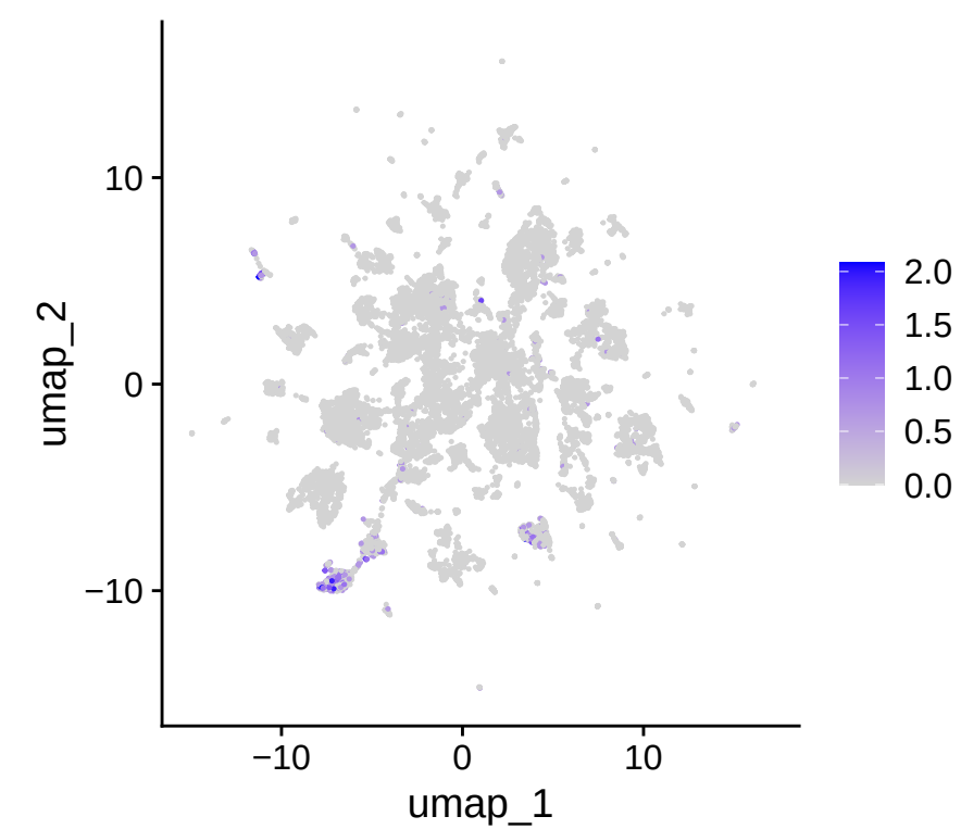
ICOS
