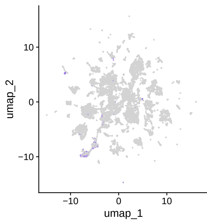
CD40LG
