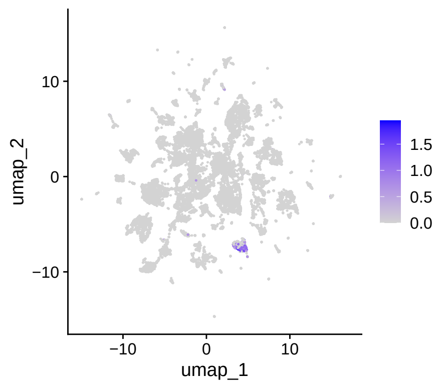
SLAMF6
