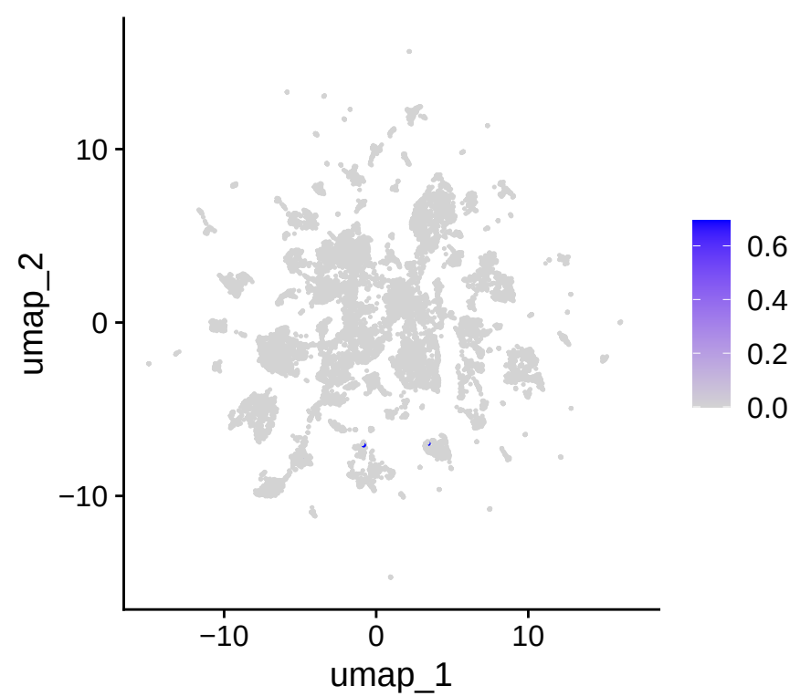
MAF
