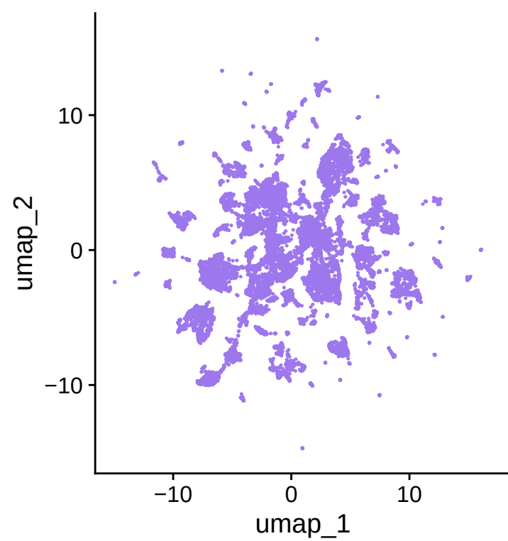
CD200
