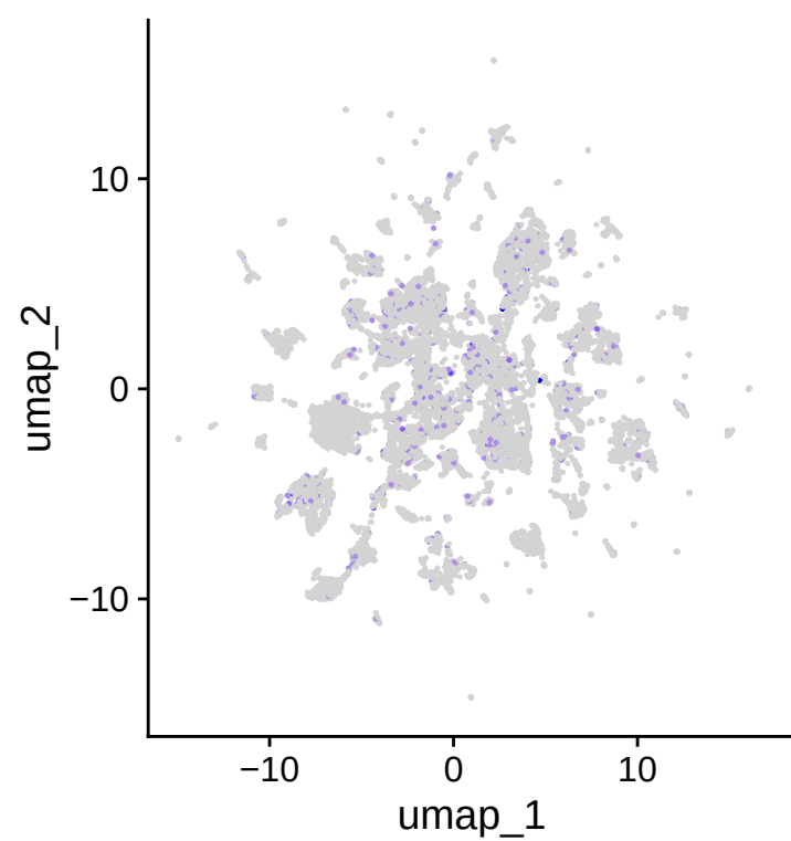
RORA
