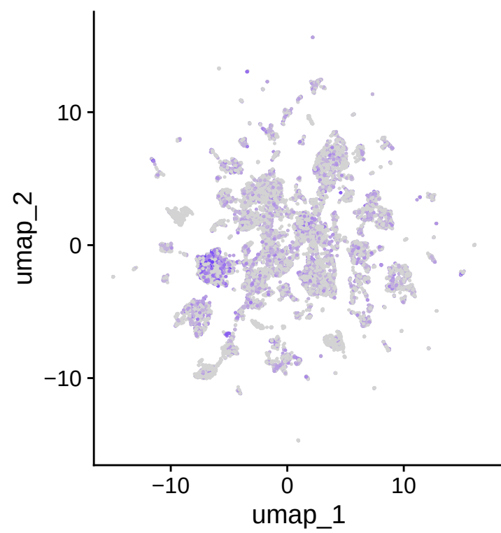
RORA
