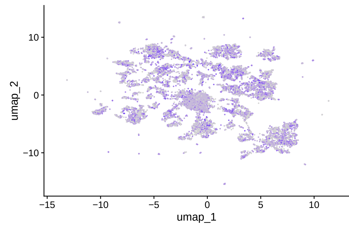
IL4R
