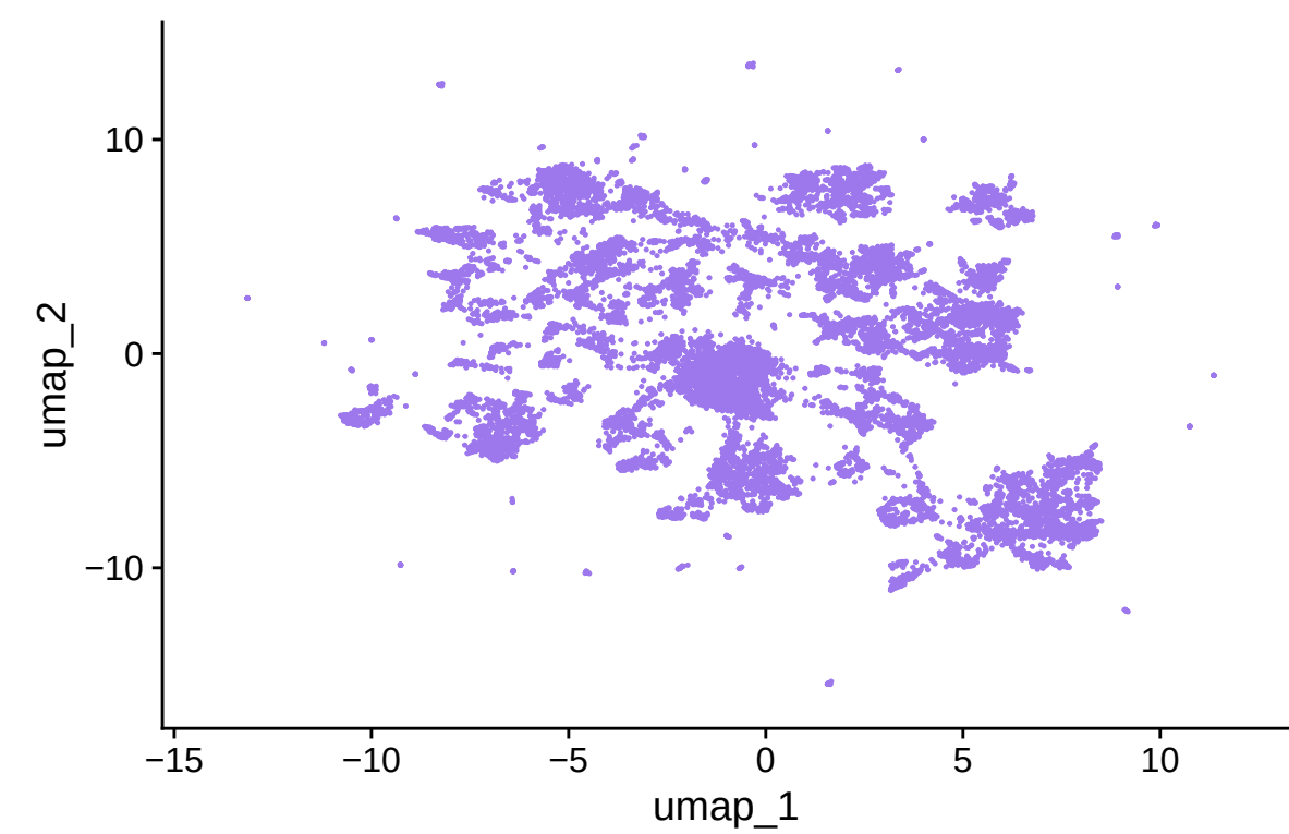
TXNIP
