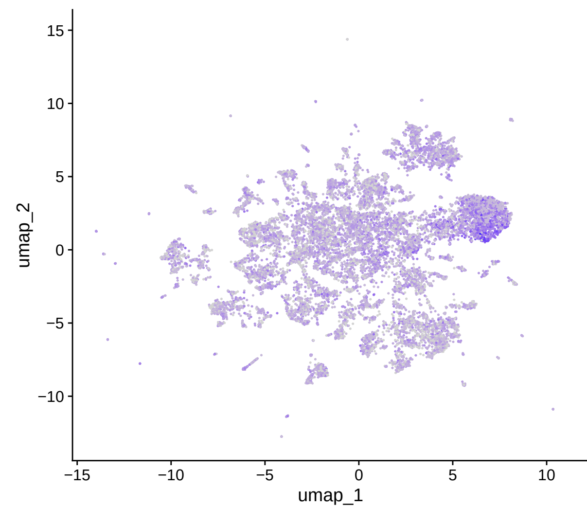
VIM
