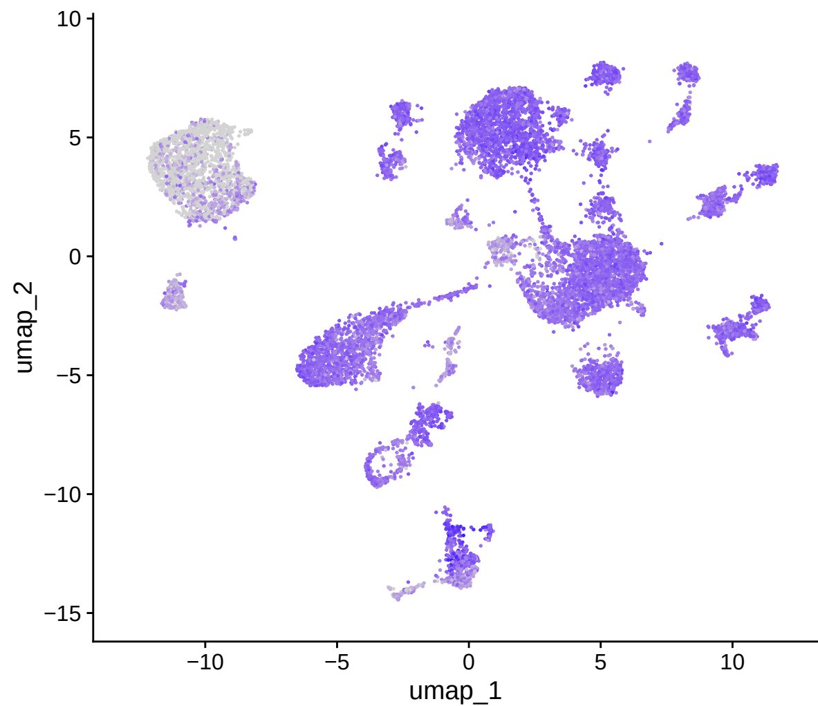
MS4A1
