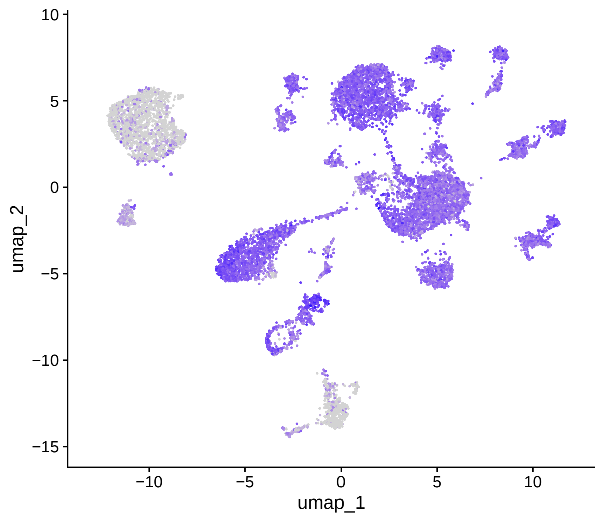
MS4A1
