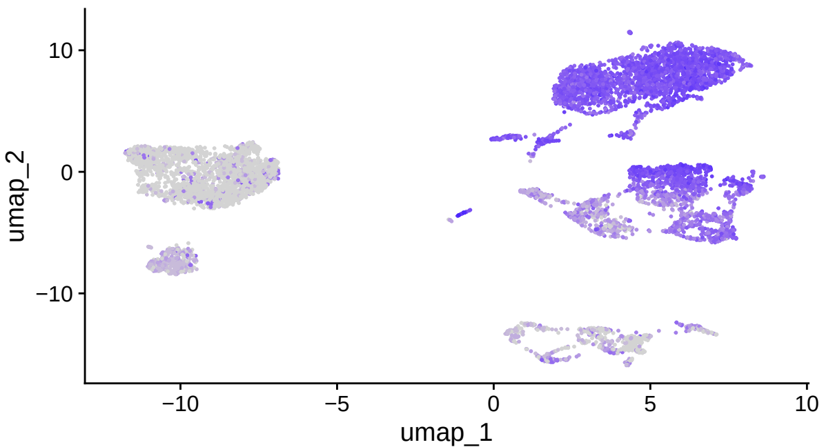
HLA-DPA1
