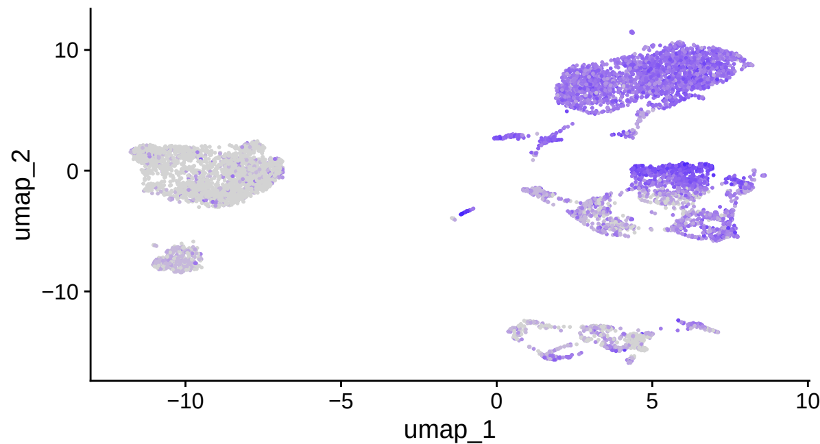
ITGAX
