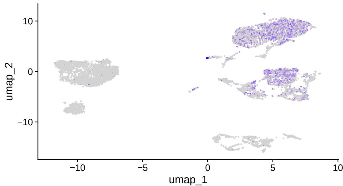
CD86
