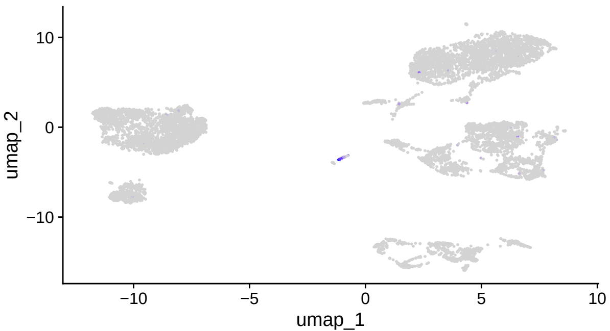
LYZ
