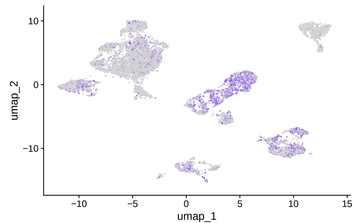
CXCR4
