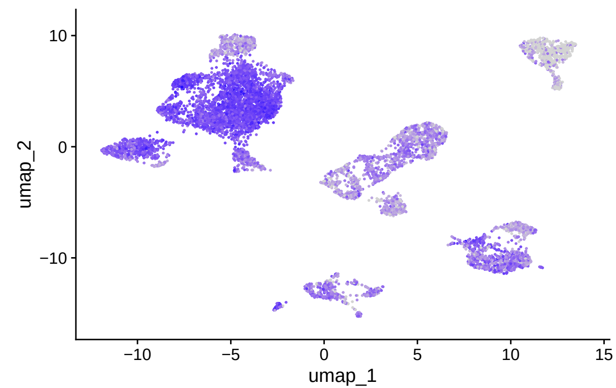
CD83
