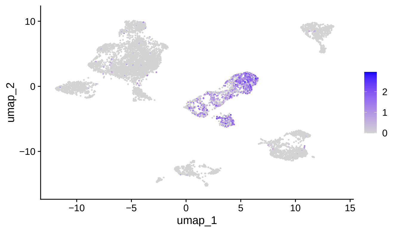
SERPINA9
