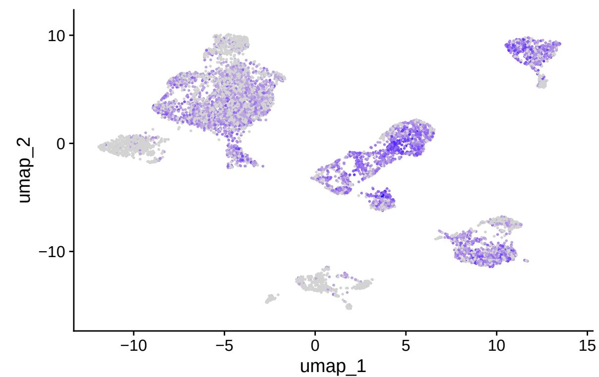
CD27
