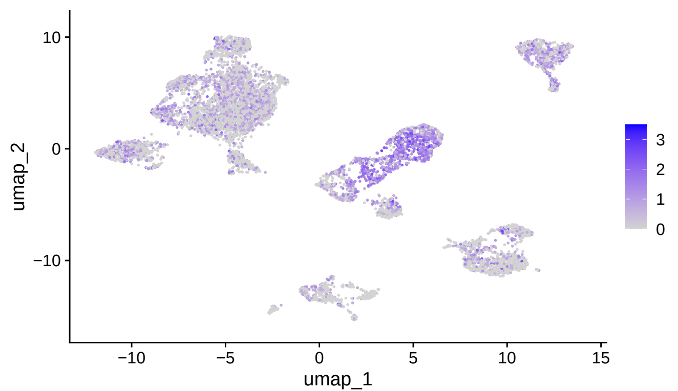
SERPINA9
