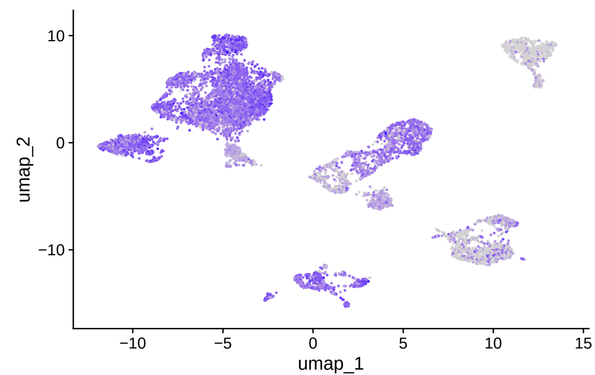
CD27
