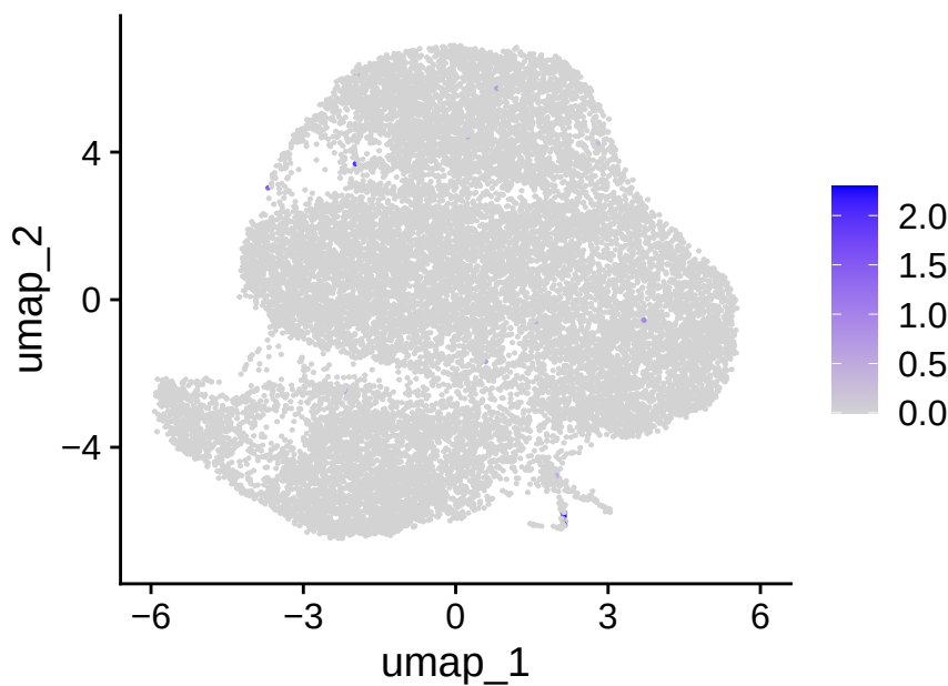
TRBC1
