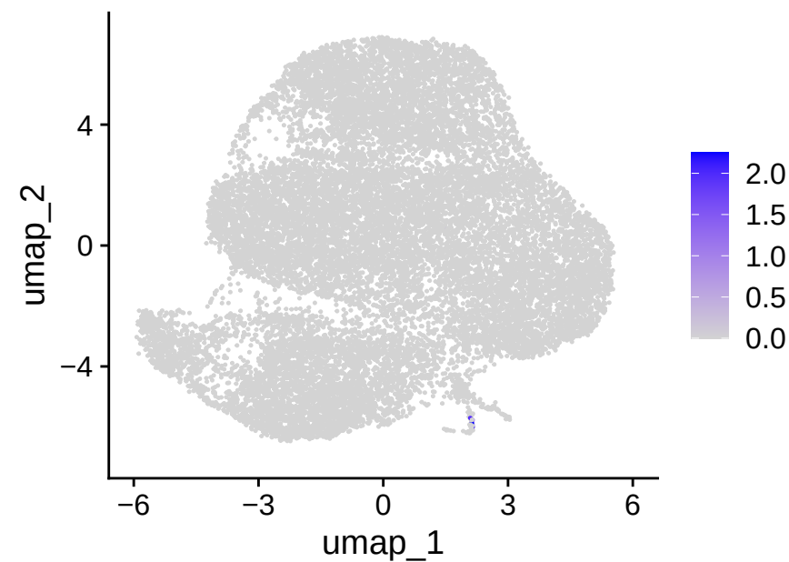
CD2
