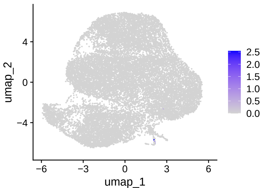
CD8A
