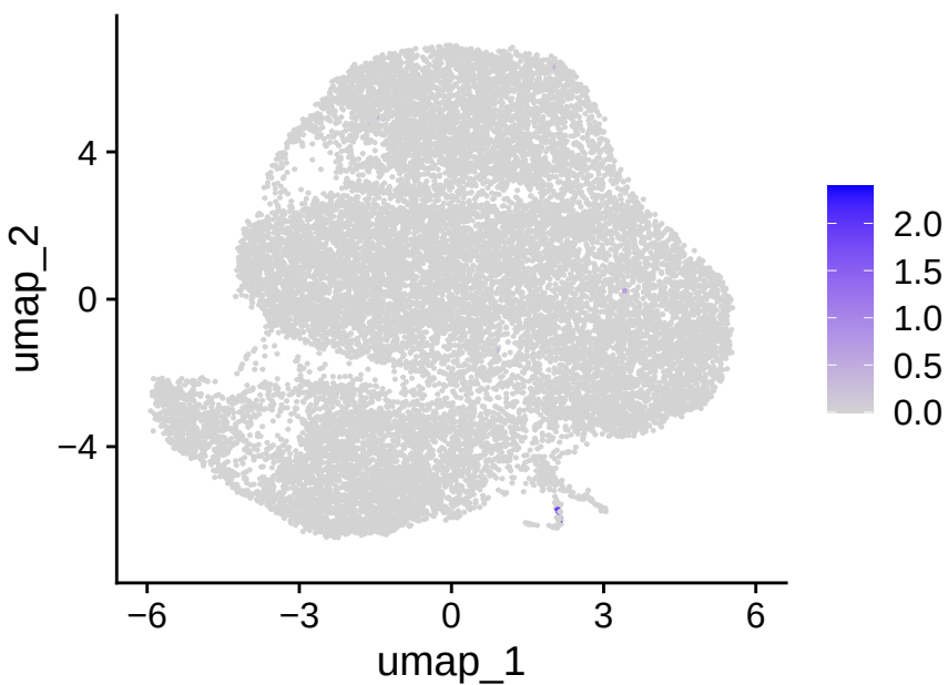
CD4
