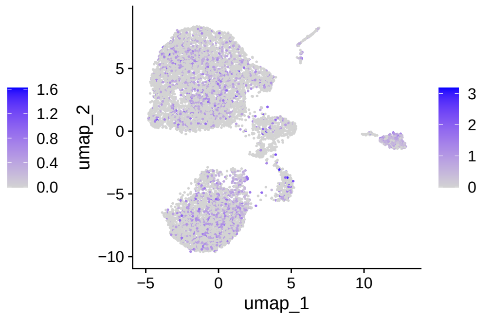
LMO2
