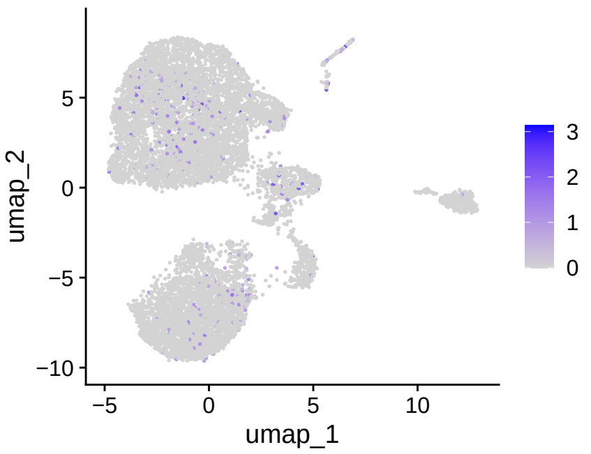
CD83
