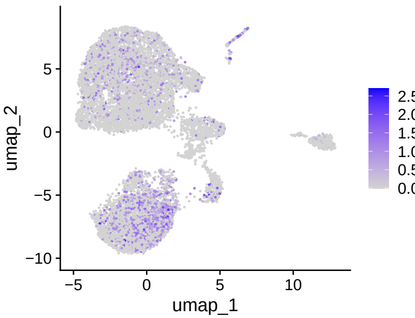
CD27
