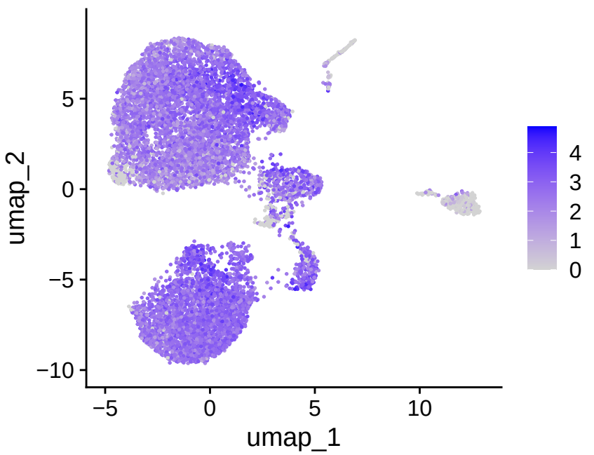
CD83
