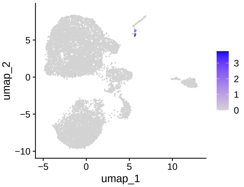
MME
