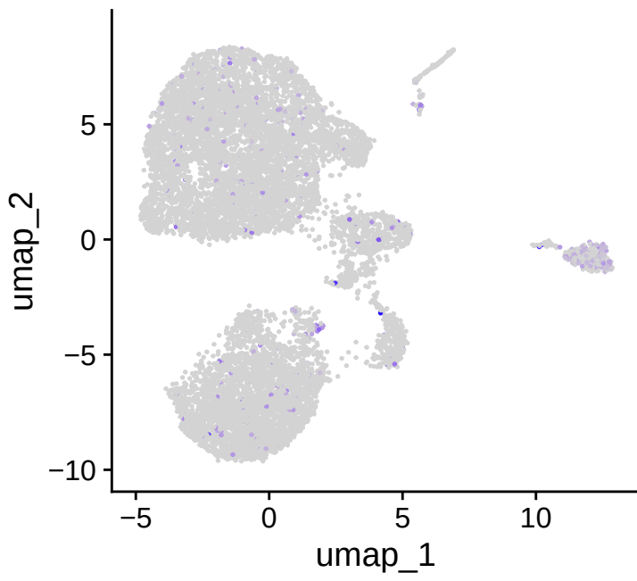
PCNA
