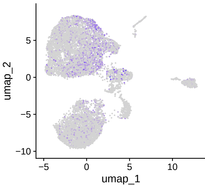
CD86
