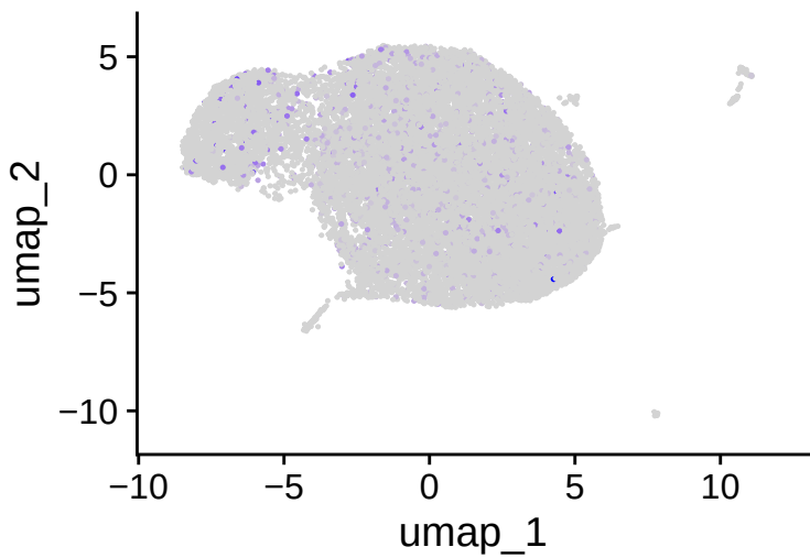
FLT3
