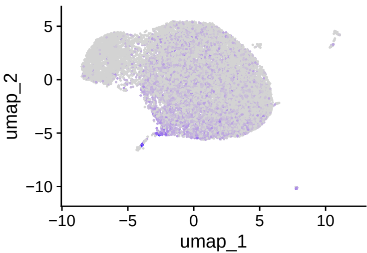
ITGAX
