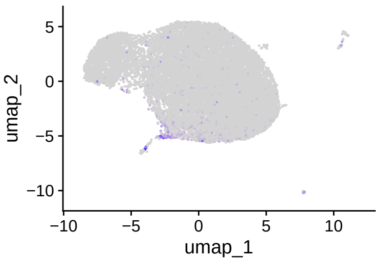
CD86
