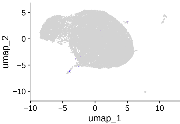
LYZ
