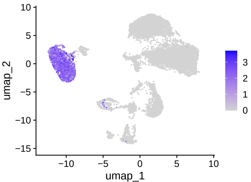
CD4
