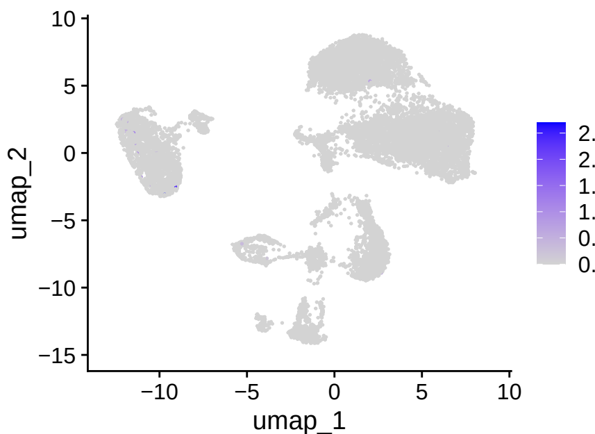
CD8A
