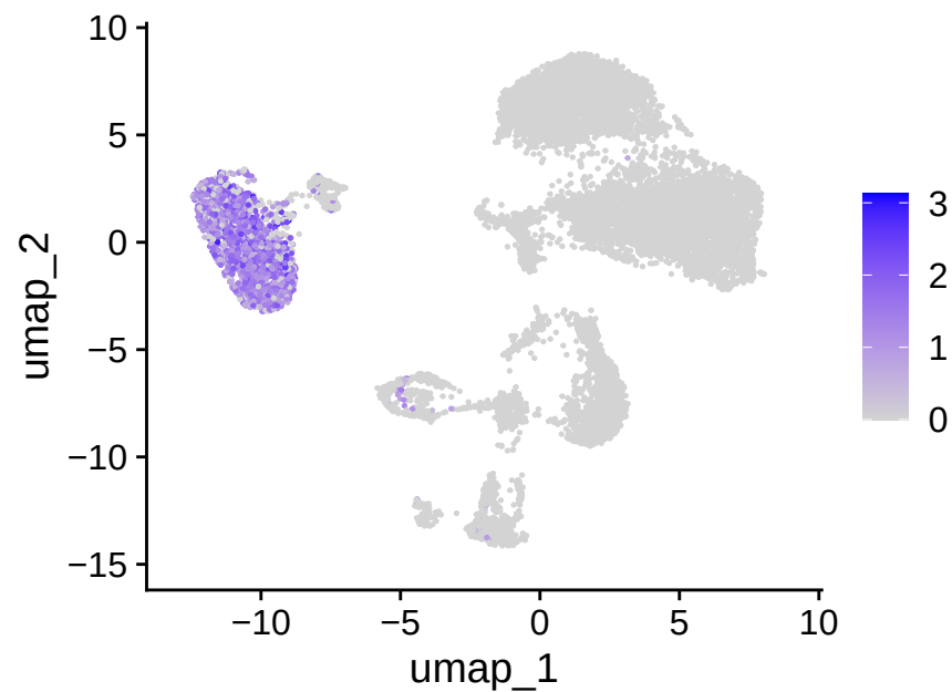
CD2
