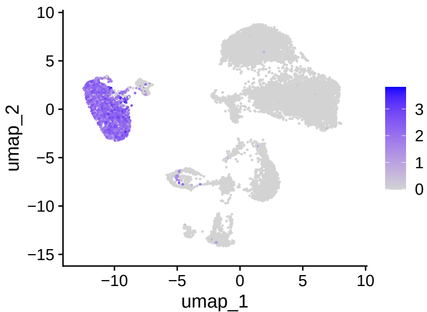
TRBC1
