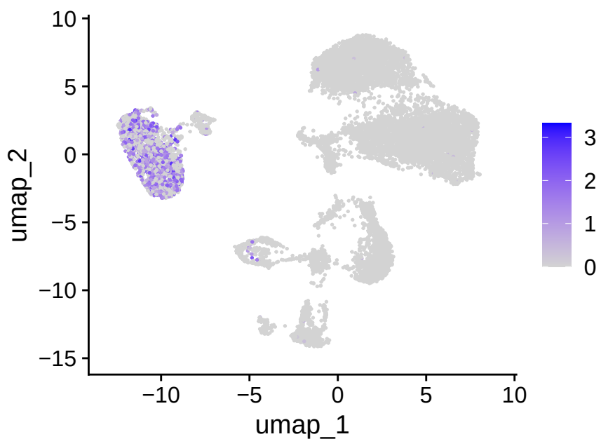
CD8A
