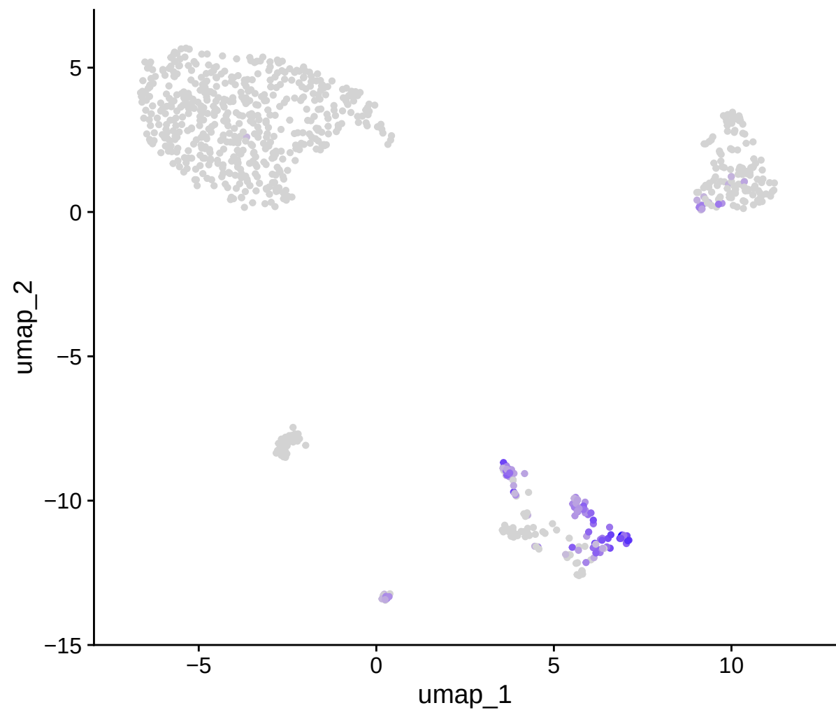
ITGAX
