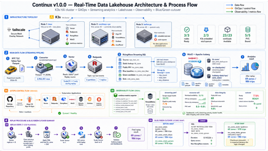
Hình 3.1: Kiến trúc và luồng quy trình Continux.
