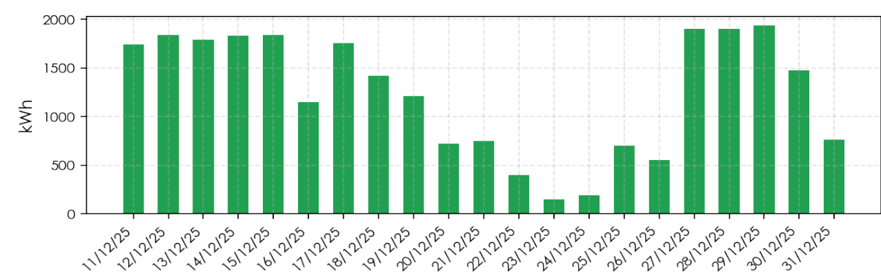
Διάγραμμα Ημερήσιας Παραγωγής (kWh)
