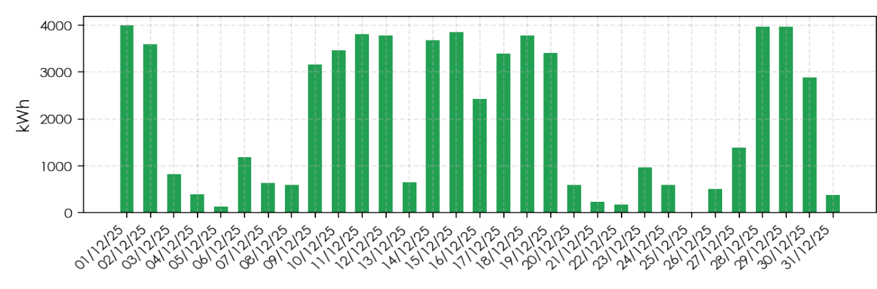
Διάγραμμα Ημερήσιας Παραγωγής (kWh)
