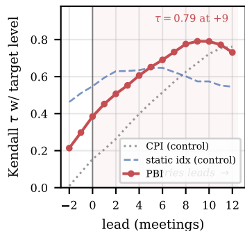
(d) the PBI leads the rate level
