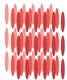
甲 结晶态
