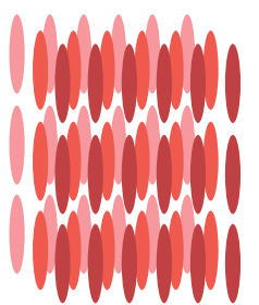
甲 结晶态
