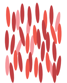
乙 液晶态
