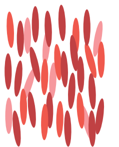
乙 液晶态
