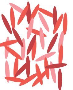
丙 液态
