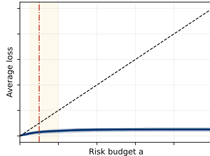
Bin 5 (n=800)
