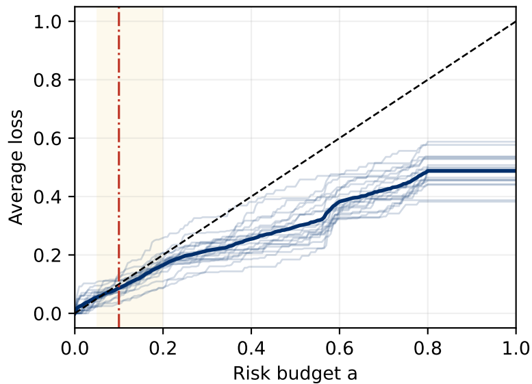
Bin 3 (n=33-107)
