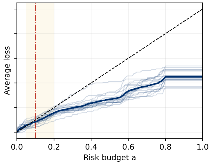
Bin 4 (n=73-127)
