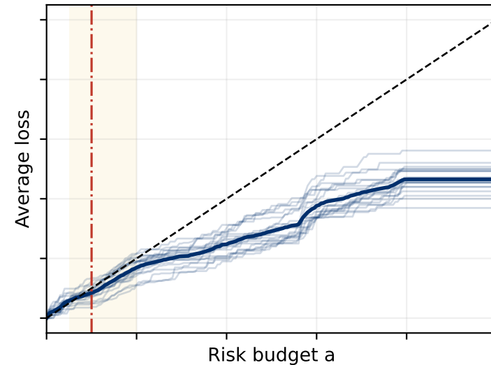
Bin 5 (n=81-88)
