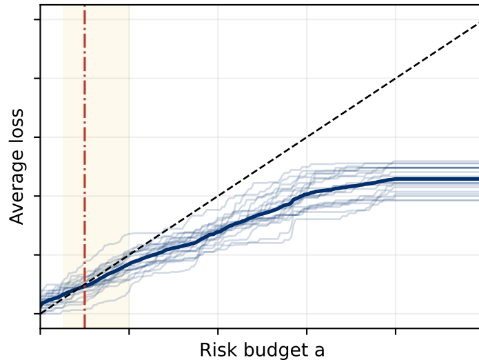
Bin 4 (n=73-127)
