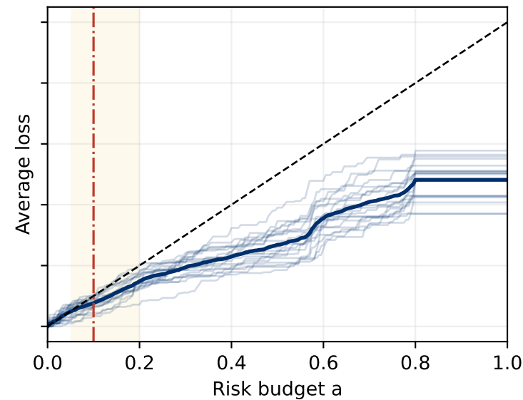
Bin 5 (n=81-88)
