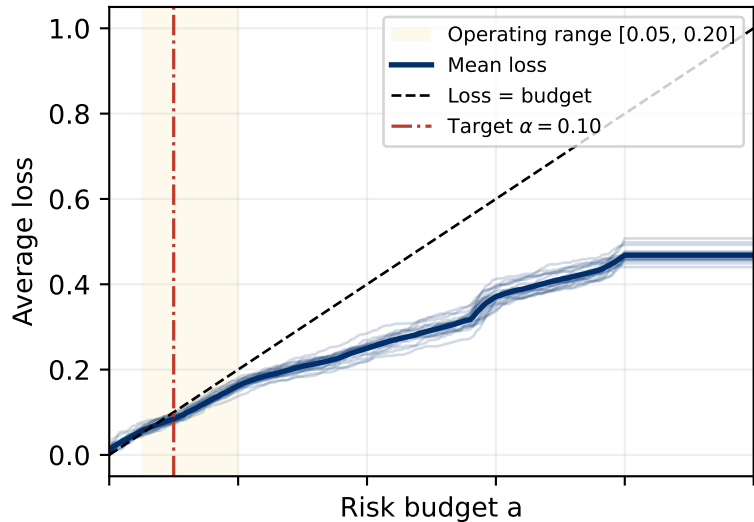
Bin 3 (n=33-107)
