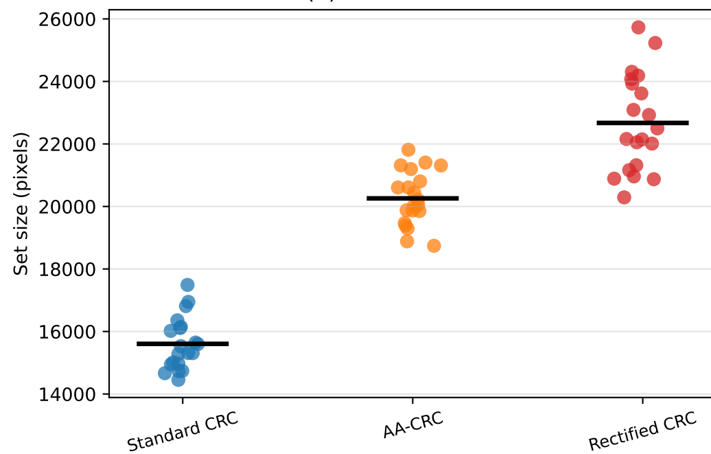
(d) Mean mask size
