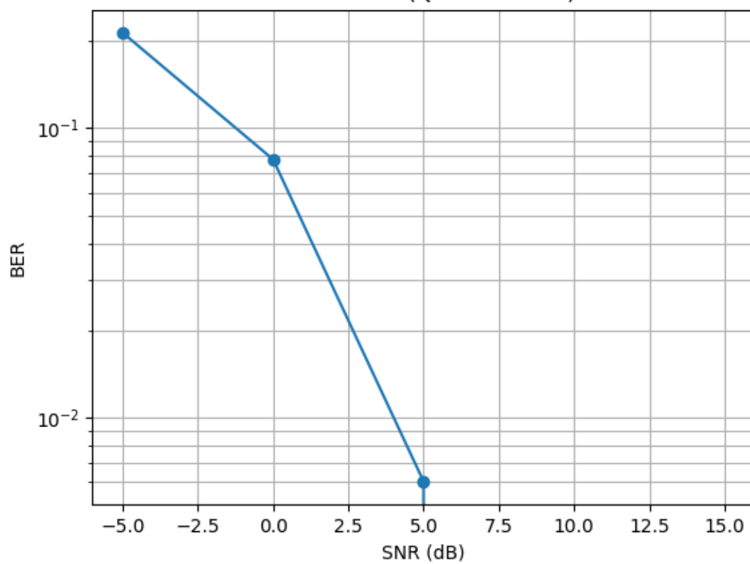
BER vs SNR (QPSK - AWGN)
