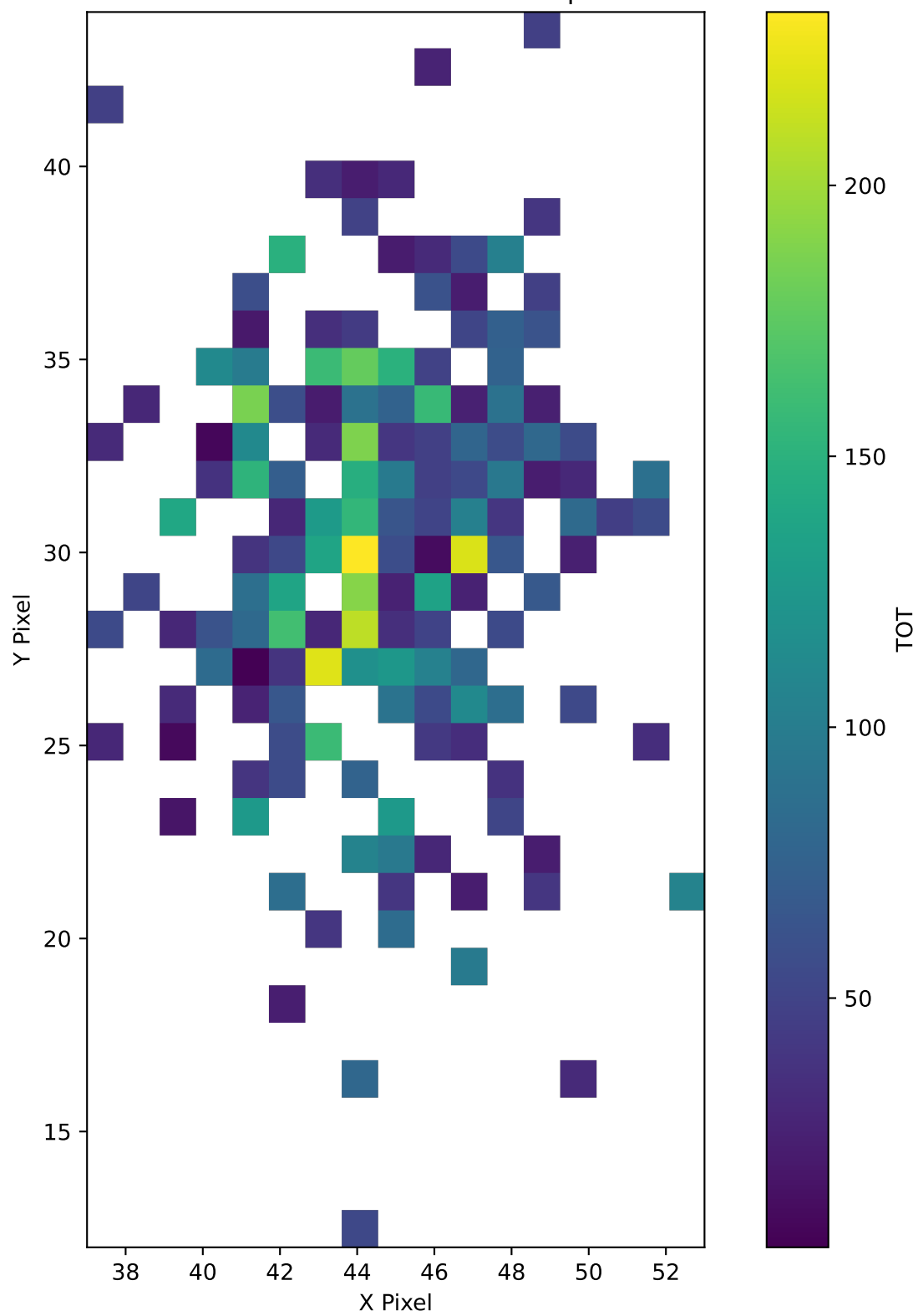
TrkID-858421 TOT Pixel Map
