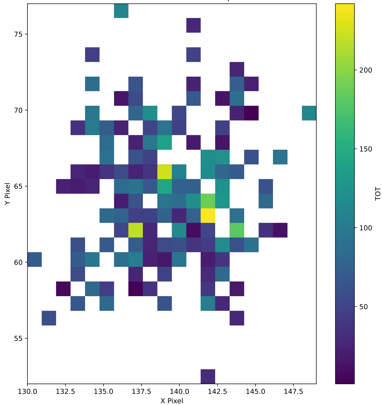
TrkID-2543115 TOT Pixel Map
