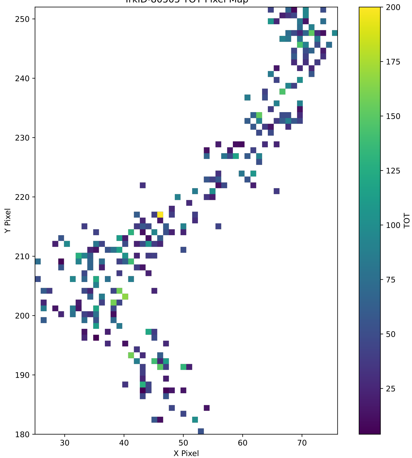
TrkID-80505 TOT Pixel Map
