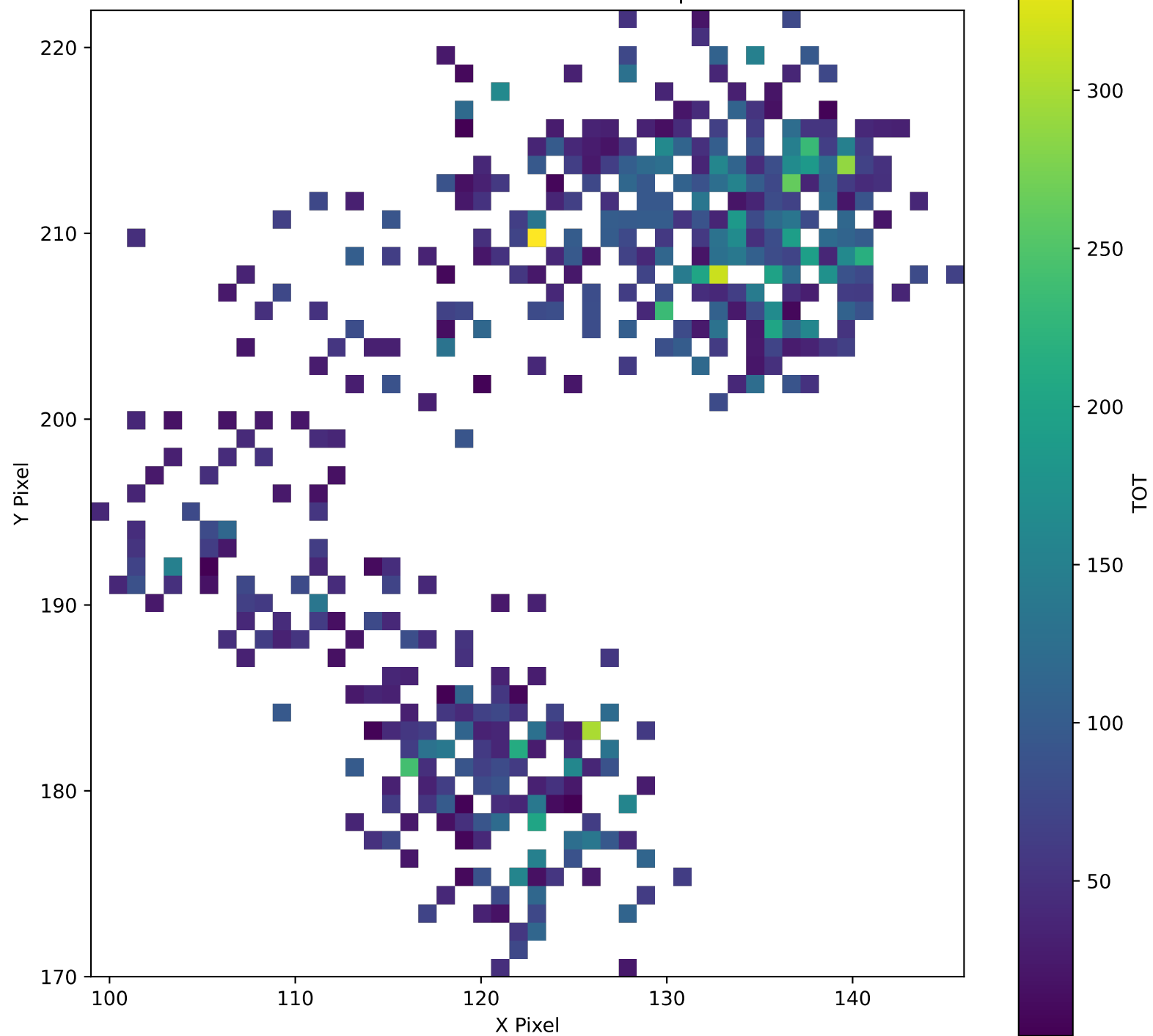
TrkID-603083 TOT Pixel Map
