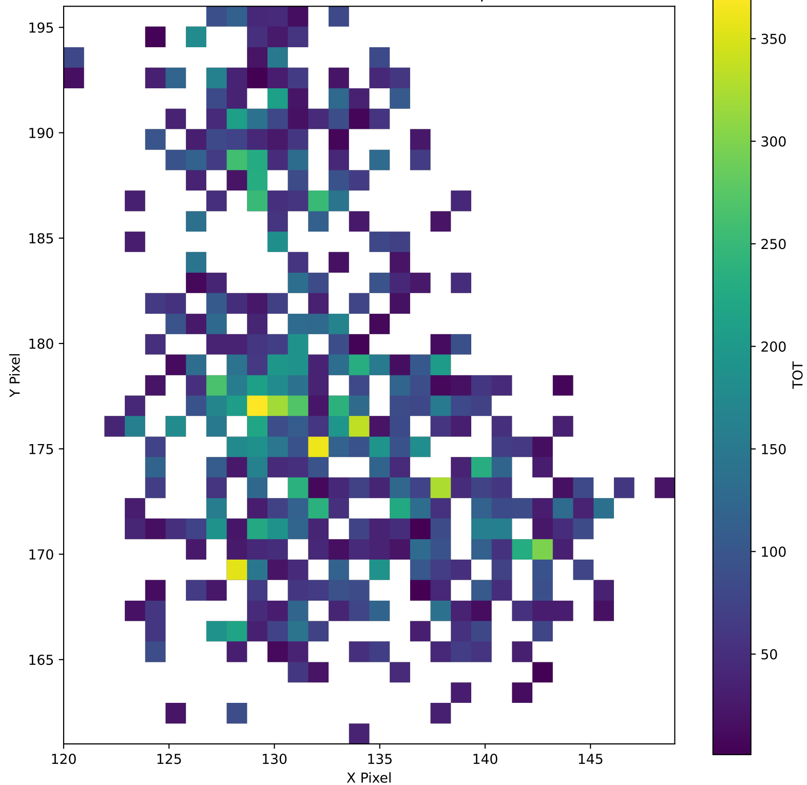
TrkID-1326932 TOT Pixel Map
