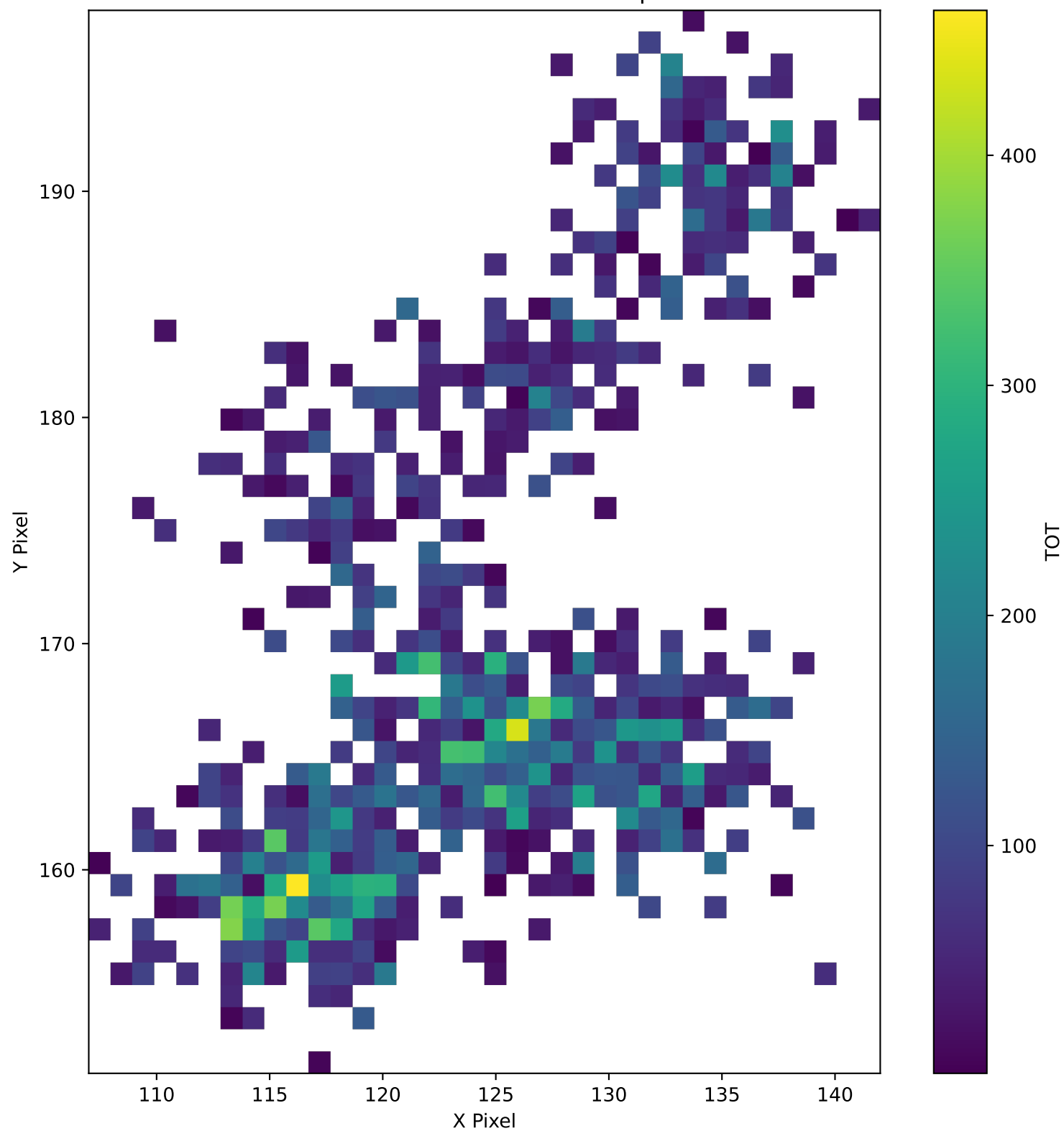
TrkID-3811249 TOT Pixel Map
