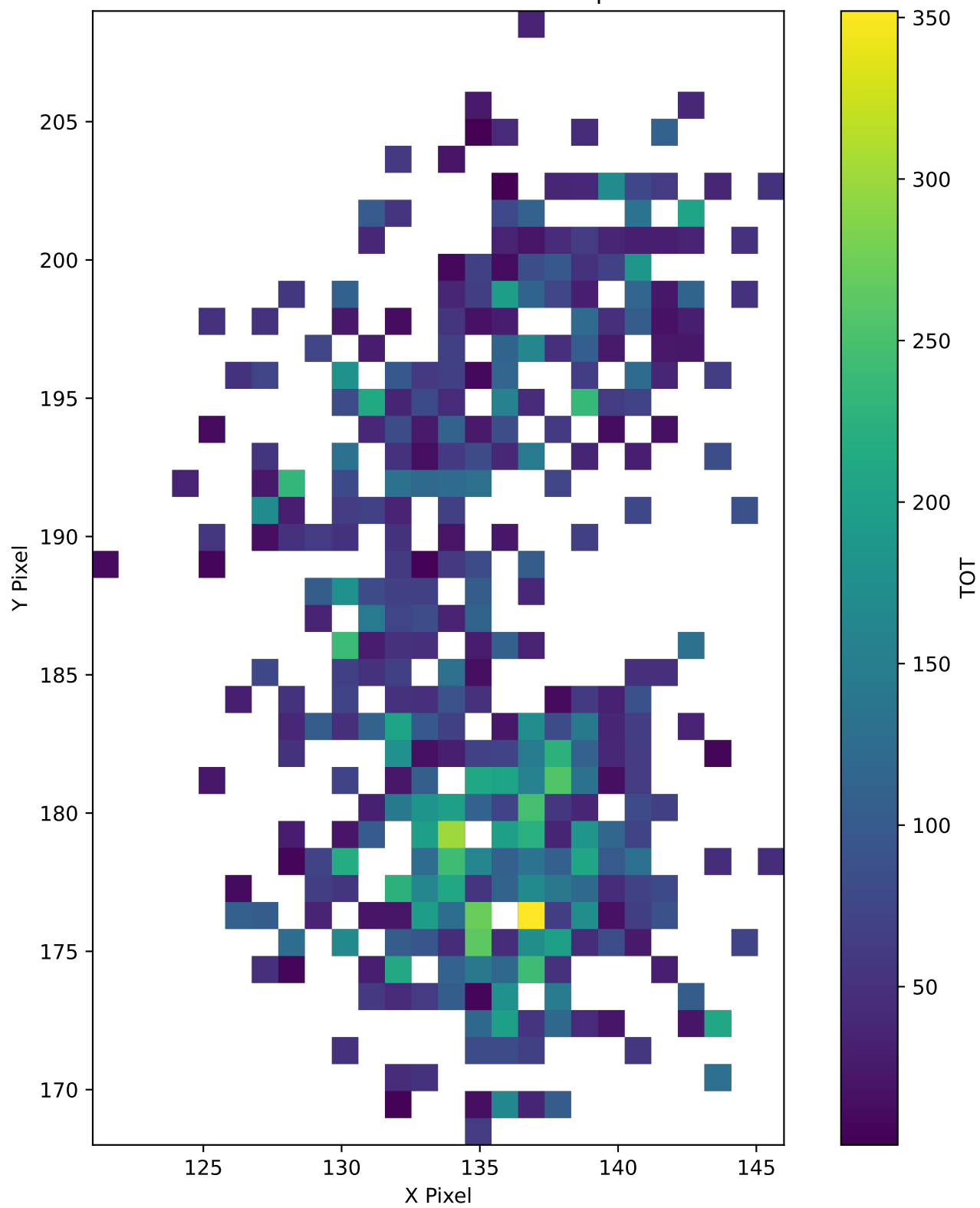
TrkID-673122 TOT Pixel Map
