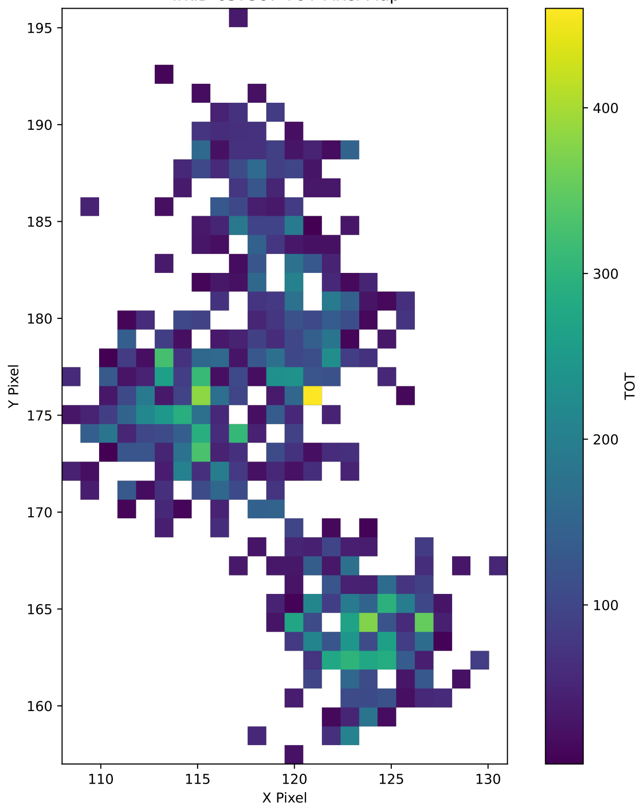
TrkID-857587 TOT Pixel Map
