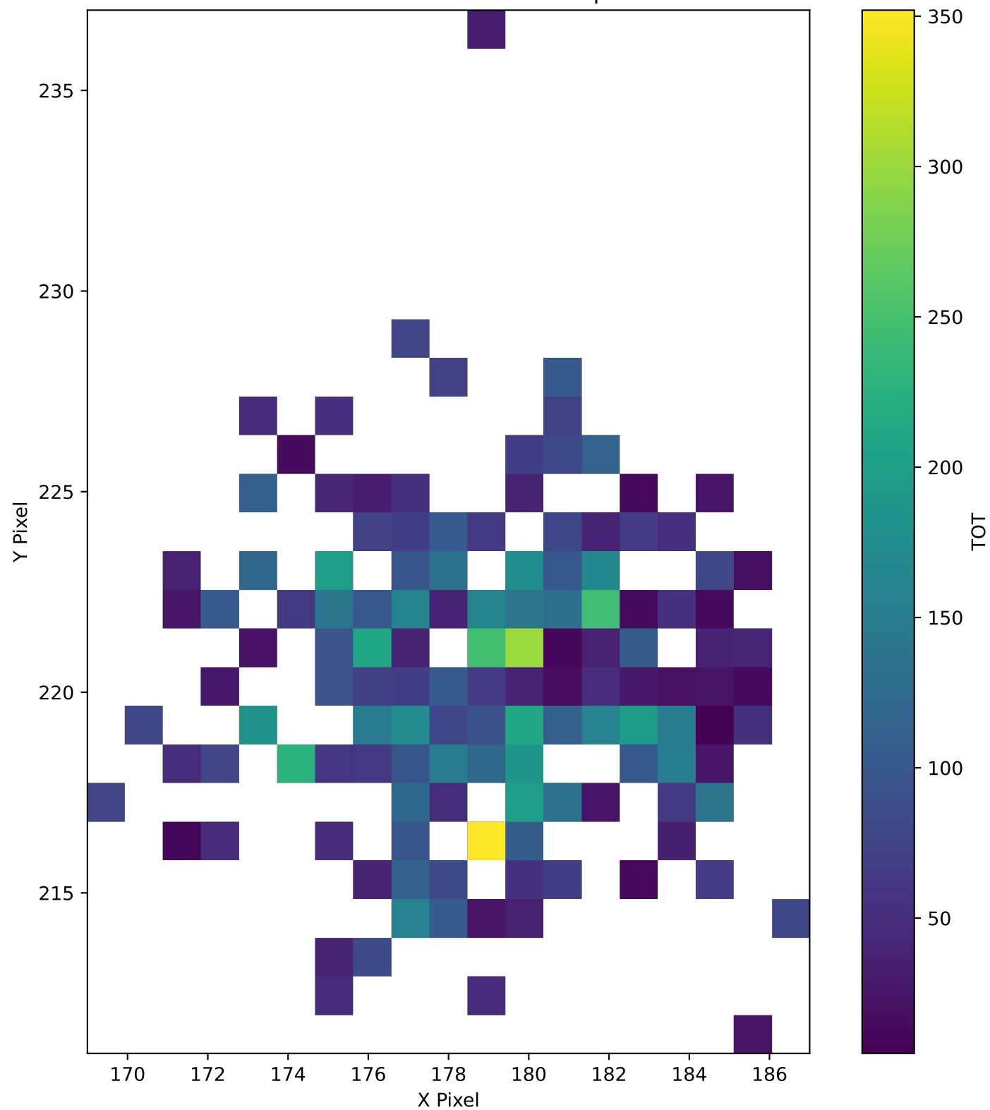
TrkID-459592 TOT Pixel Map
