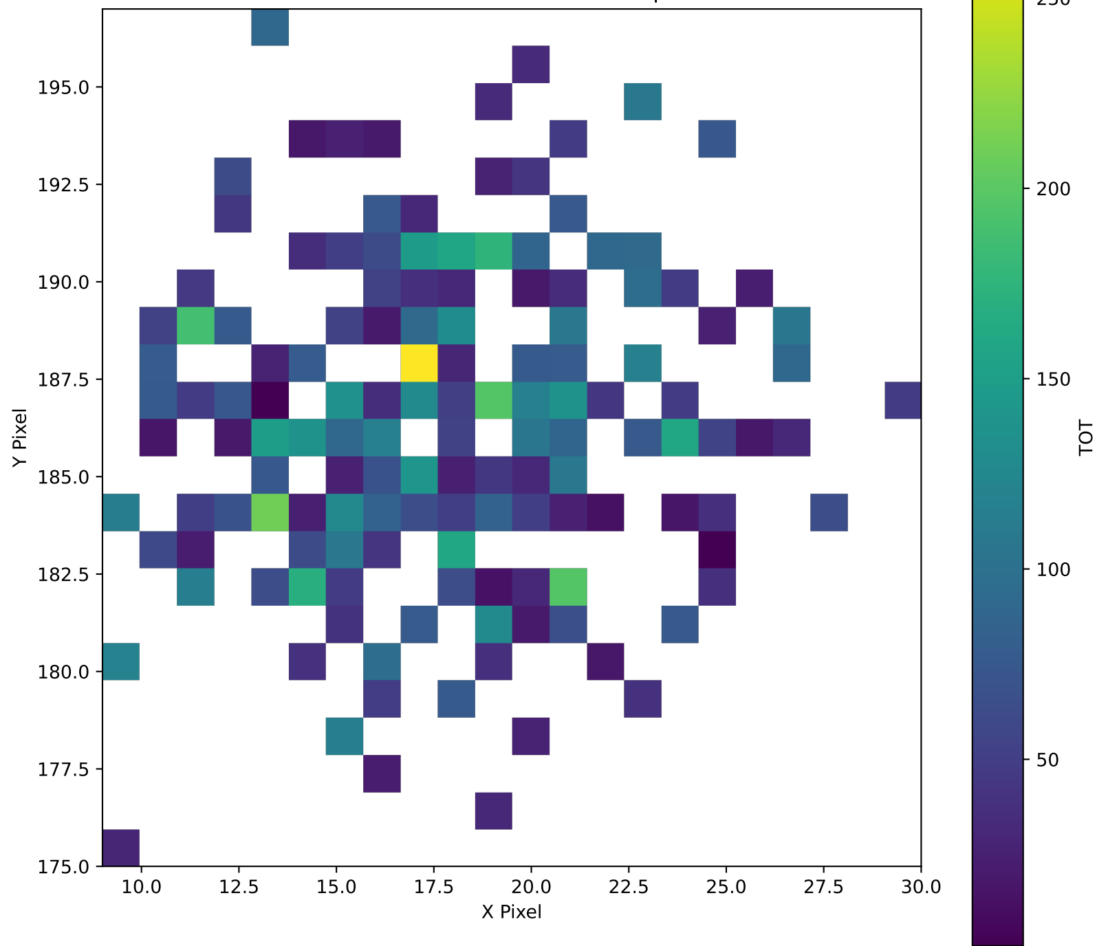
TrkID-236791 TOT Pixel Map
