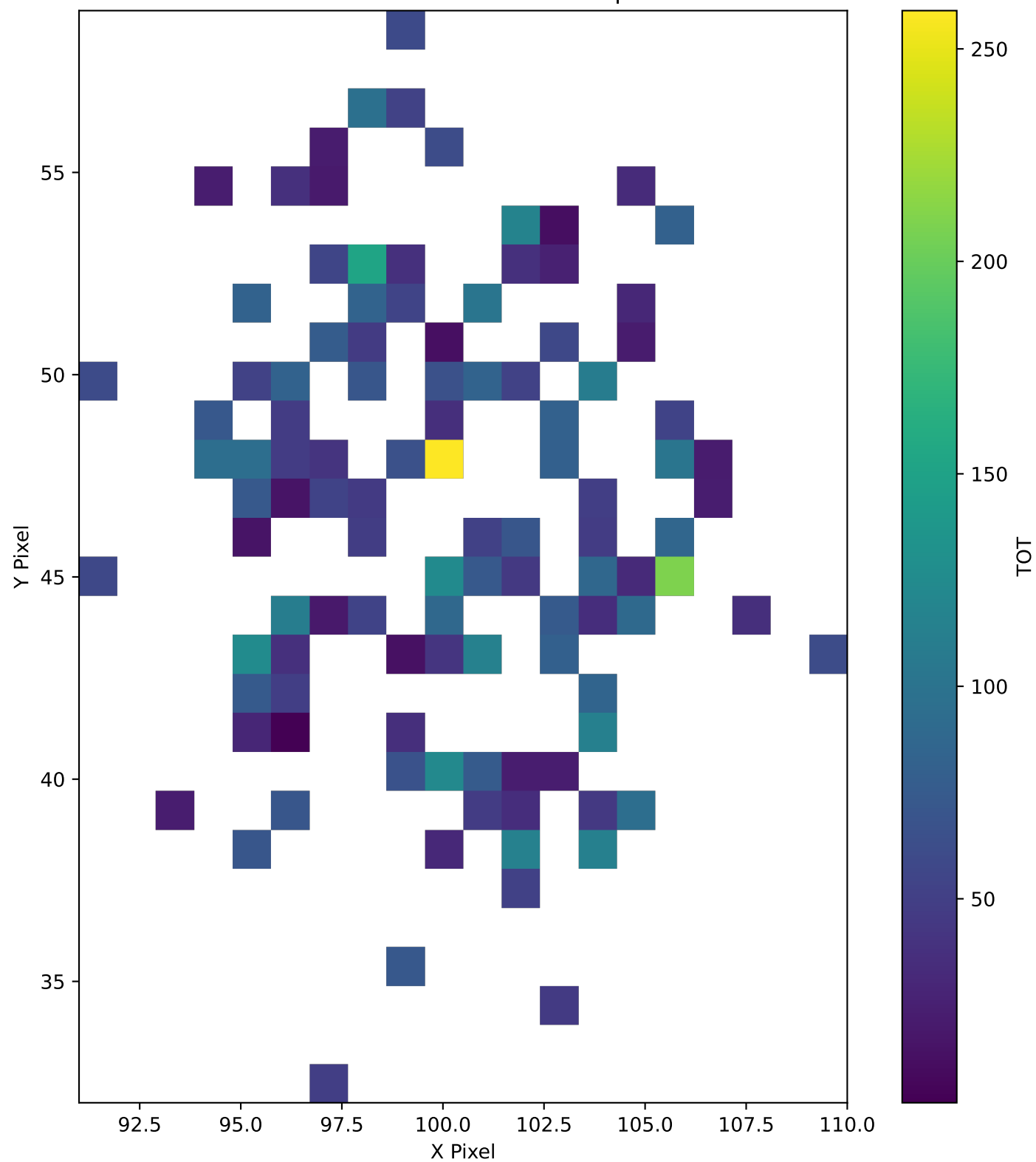
TrkID-445112 TOT Pixel Map
