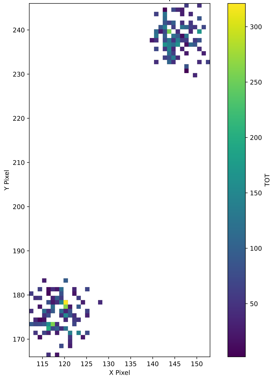
TrkID-558632 TOT Pixel Map
