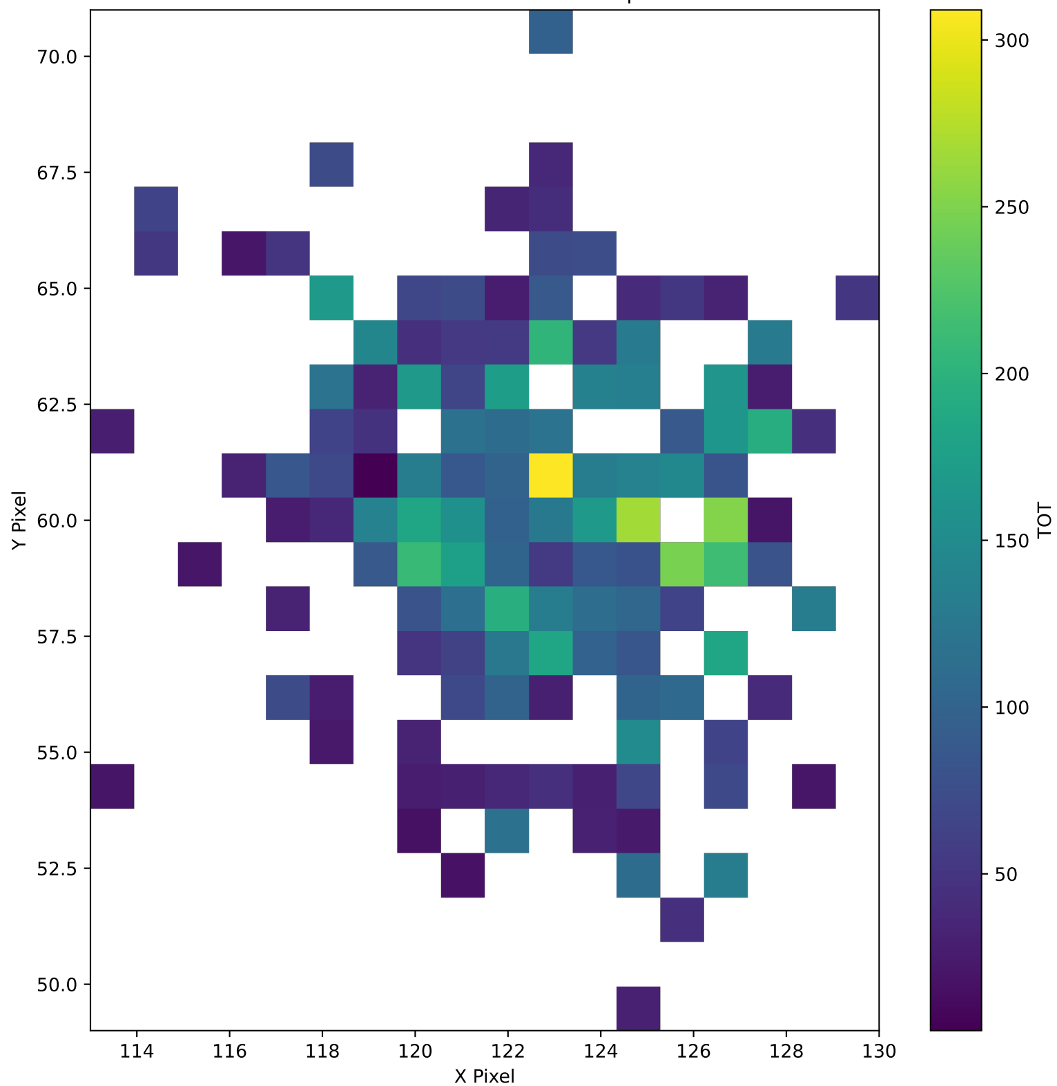
TrkID-586595 TOT Pixel Map
