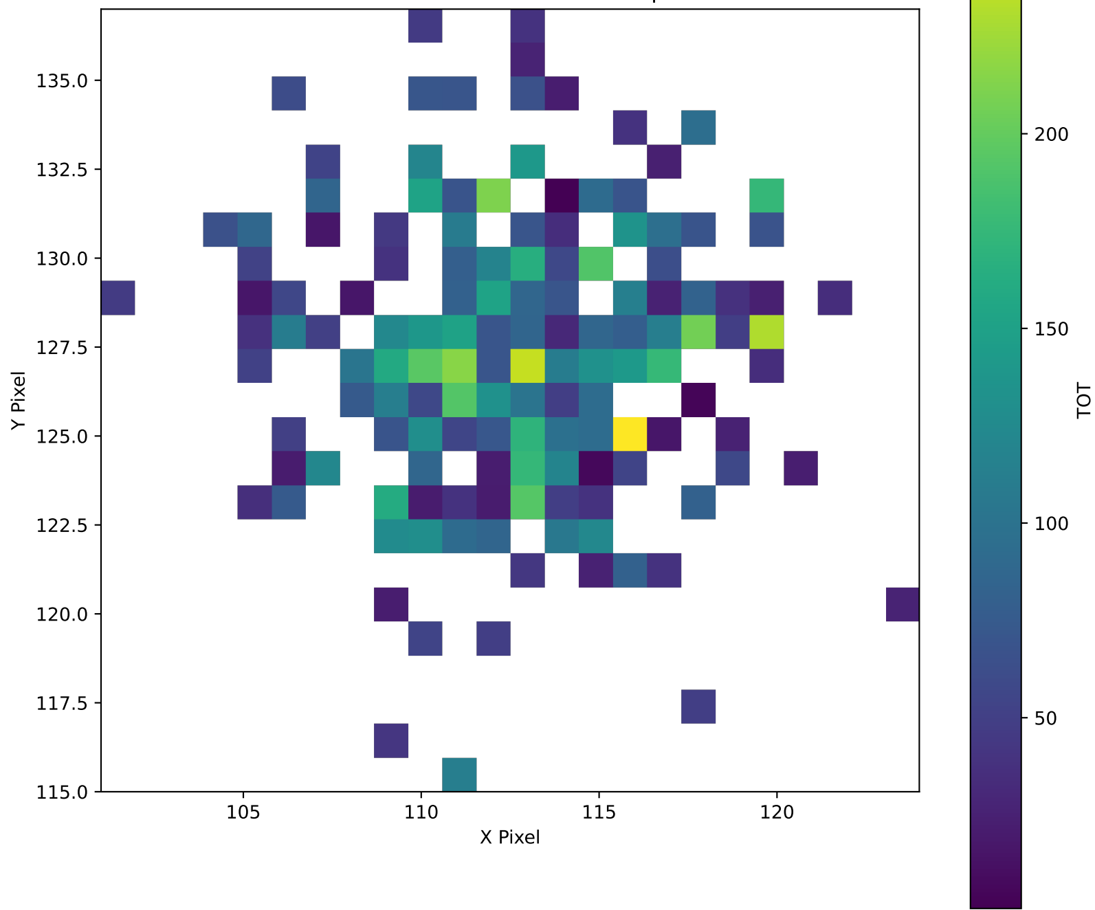
TrkID-592916 TOT Pixel Map
